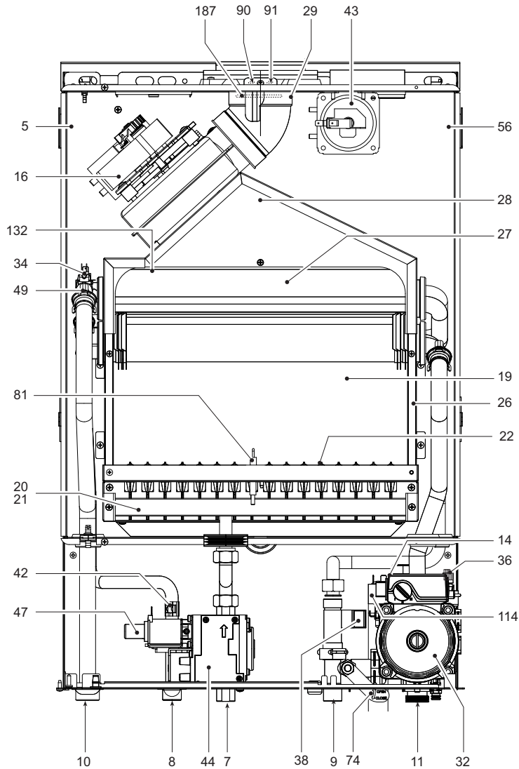
рис. 20 - Общий вид
