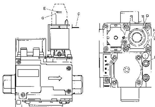
рис. 16 - Газовый клапан
