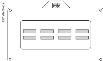
2 шины 50 x 10
