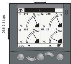
Дисплей FDM121: значения токов
