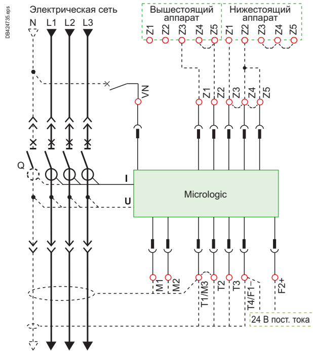
Маркировка клемм
