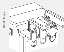
Расширители полюсов
