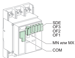
Аппараты с электрическим управлением
