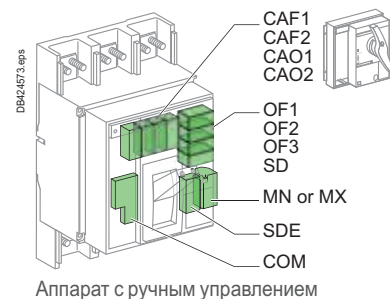
Аппарат с ручным управлением
