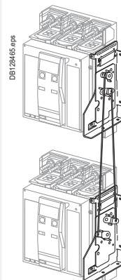
Взаимоблокировка штангами
