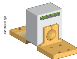
Внешний ТТ (ТСЕ)
