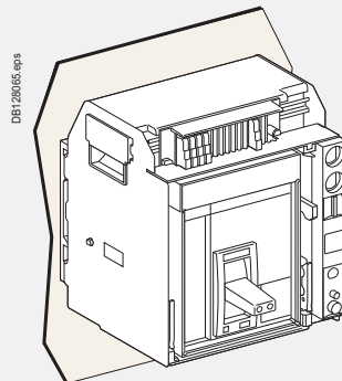
Заднее крепление на панели
