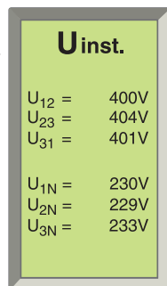
Индикация напряжений
