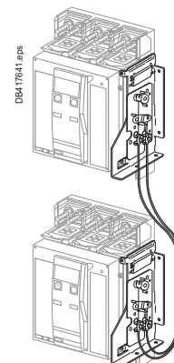
Взаимоблокировка тросовыми тягами
