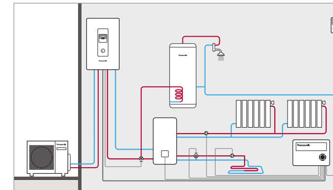
Управление температурой в 2 зонах + ECS с PAW-HPM12ZONE-U
