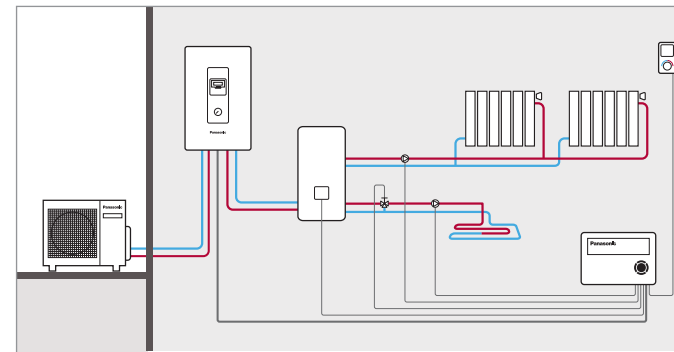
Управление температурой в 2 зонах с PAW-HPM12ZONE-U
