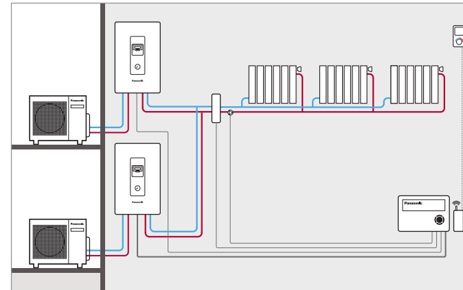
2 тепловых насоса, управляемых в каскадном режиме, с PAW-HPM12ZONELCD-U
