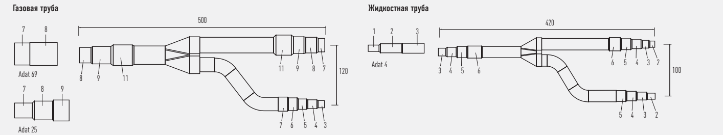
Габаритные размеры: мм
