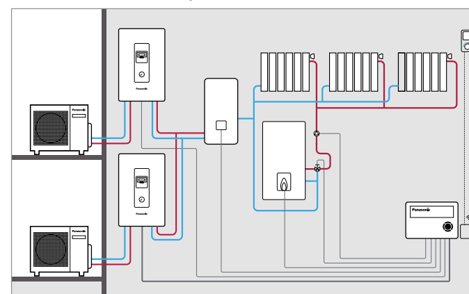
2 тепловых насоса + бойлер с PAW-HPM12ZONE-U
