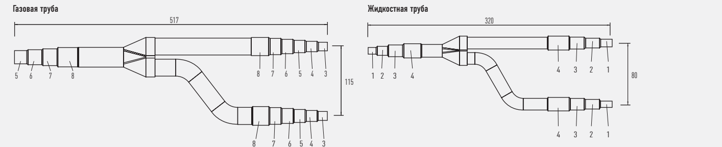
Габаритные размеры: мм
