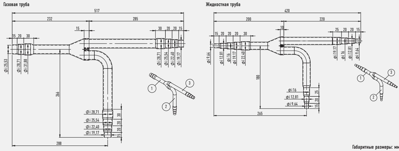
Габаритные размеры: мм
