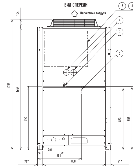
*Монтажный кронштейн, сторона крепления.
