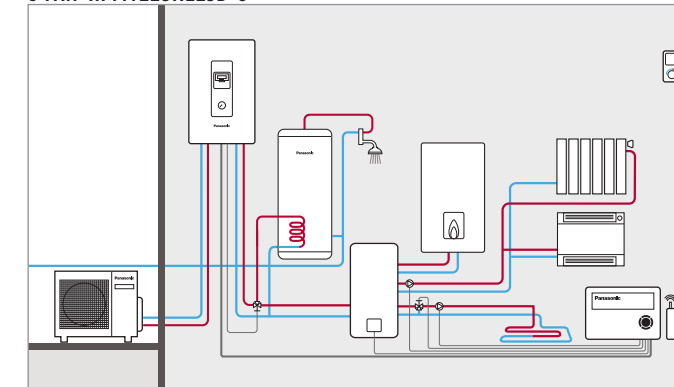
Управление тепловым насосом + бойлер и система DHW с PAW-HPM12ZONELCD-U
