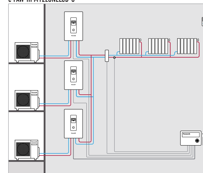
3 тепловых насоса, управляемых в каскадном режиме, с PAW-HPM12ZONELCD-U
