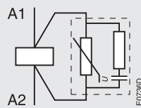
Варистор + RC-цепочка
