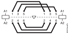
Соединительный комплект BEM... E0744D
