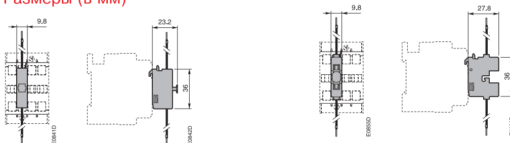
Блоки патронов для ламп BL 5-L Блоки патронов для плавких вставок BL5-F
