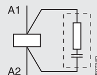
RC цепочка
