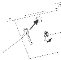
Der „Wassertank voll“ - Absperrschalter ist niedergedrückt, wenn das Ablaufrohr für kontinuierliche Entwässerung befestigt ist.
