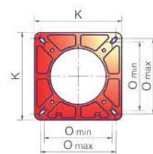
Фланец горелки
