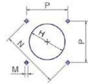
Рекомендуемая амбразура котла
