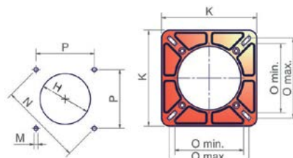
Рекомендуемая амбразура котла
