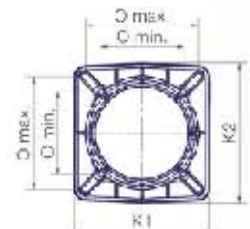
Фланец горелки
