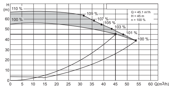
Рис. 108 Пример расширенного диапазона производительности до 110 % в рамках рабочего диапазона
