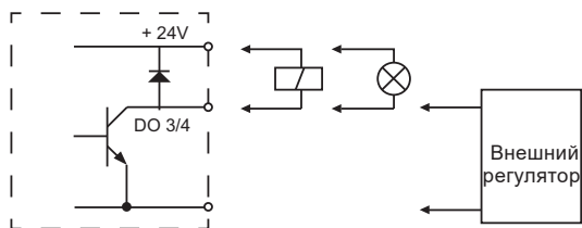
Рис. 137 Пример настраиваемых цифровых входов или выходов
