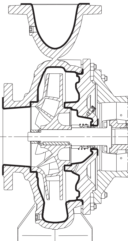
Рис. 87 Вид в разрезе насоса с покрытием для морской воды до 25 °С
