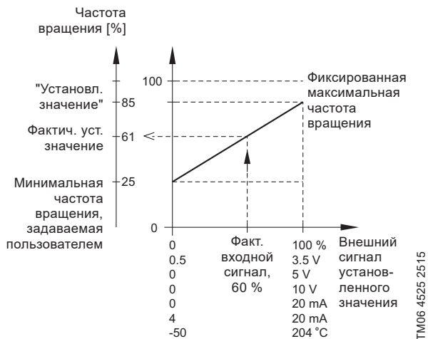
Рис. 141 Пример влияния установленного значения на постоянную характеристику
