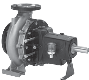
Рис. 66 Масленка постоянной смазки
