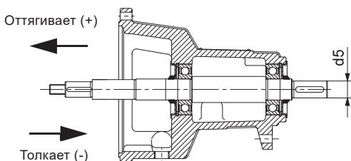
Рис. 61 Направление усилий, действующих на подшипники
