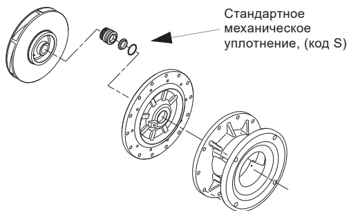
Рис. 27 Насосы NB, NBG со стандартным оди́рным уплотнением
