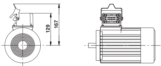
Рис. 13 Размеры, 0,37 - 1,1 кВт
