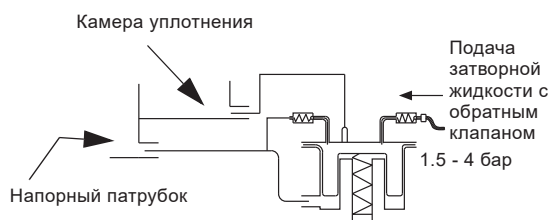
Рис. 48 Схема монтажа соединений гидромultiпликатора
