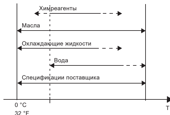
Рис. 34 Диапазон рабочих температур механического уплотнения вала для различных категорий жидкостей по сравнению со спецификациями поставщиков.
