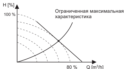
Рис. 133 Ограничения по мощности и давлению, влияющие на максимальную характеристику
