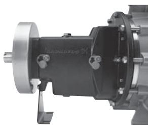
Рис. 68 Фитинги SPM в кронштейне подшипника
