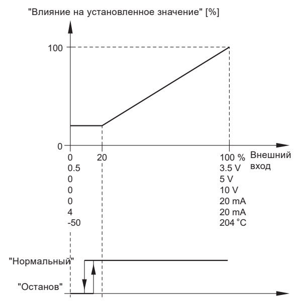
Рис. 143 Линейная функция с остановом
