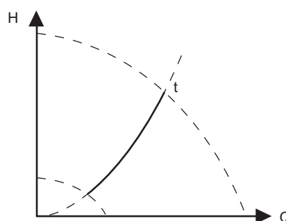
Рис. 122 "Постоянная температура"
