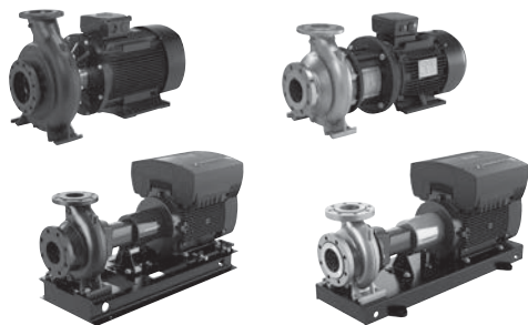
Рис. 4 Насосы NB, NBE, NBG, NBGE, NK, NKE, NKG, NKGE с датчиком
