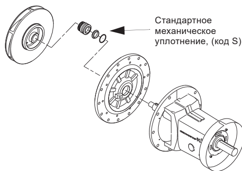
Рис. 28 Насосы NK, NKG со стандартным оди́рным уплотнением
