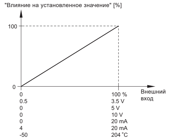
Рис. 142 Линейная функция
