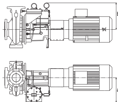
Рис. 49 Насос с гидромultiпликатором давления Указанные значения относятся к насосам NKG всех типоразмеров
