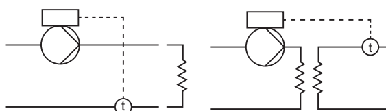
Рис. 123 "Постоянная температура"
