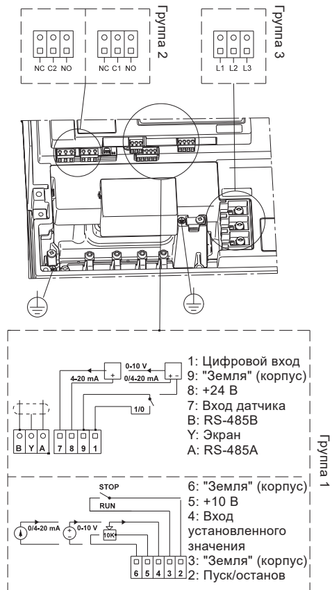
Рис. 153 Клеммы соединений
