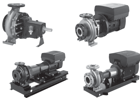
Рис. 9 Насосы NB, NBG, NK, NKG, NBE, NBGE, NKE, NKGЕ
