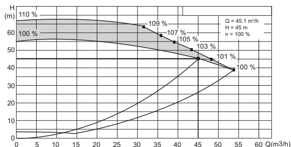
Рис. 98 Пример расширенного диапазона производительности до 110 % в рамках рабочего диапазона
