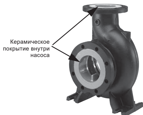
Рис. 78 Насос с керамическим покрытием
