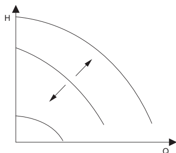
Рис. 132 "Постоянная характеристика"
