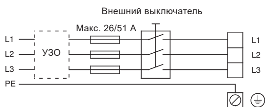
Рис. 152 Схема соединений, трехфазные электродвигатели MGE, 11-22 кВт
