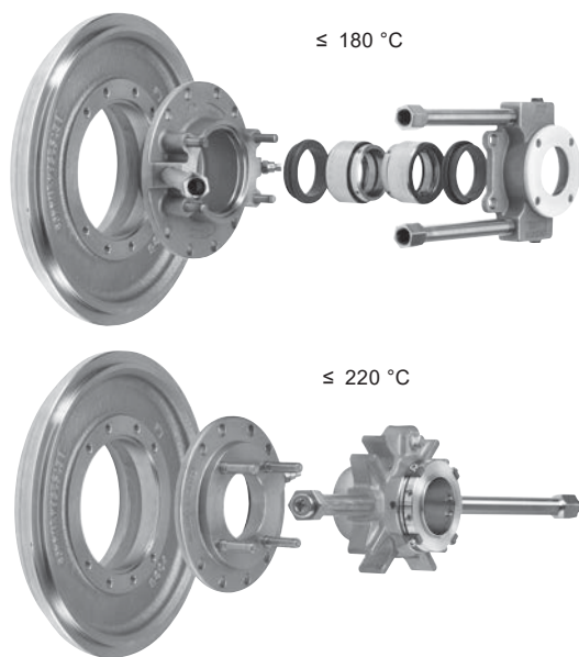
Рис. 44 Уплотнение типа "back-to-back" в качестве стандартного уплотнения или картриджного уплотнения
