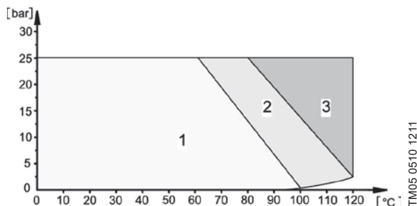
Рис. 33 Рабочие диапазоны
