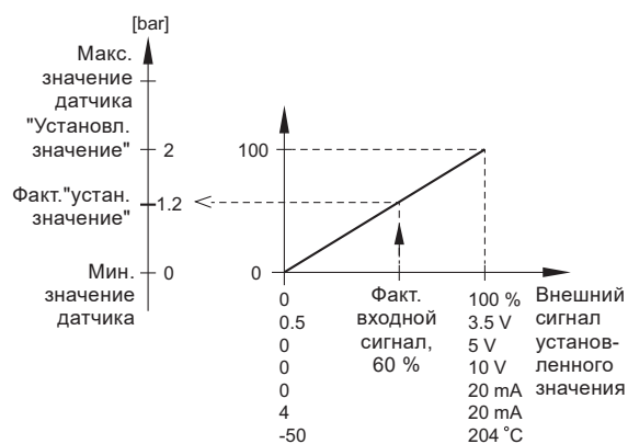
Рис. 140 Пример изменения установленного значения по сигналам с датчиков
