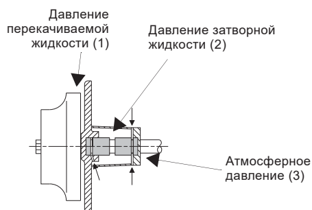
Рис. 41 Давление в уплотнении типа "back-to-back"
