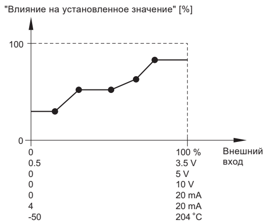
Рис. 144 "Таблица регулирования", пример с пятью точками
