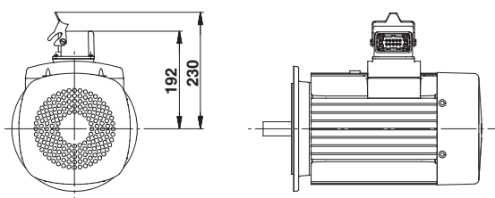
Рис. 14 Размеры, 1,5 - 7,5 кВт
