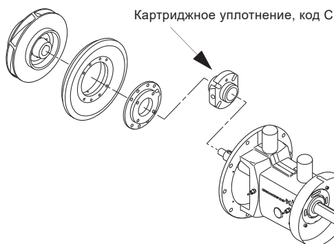
Рис. 29 Расположение картриджного оди́рного уплотнения в насосе NKG
