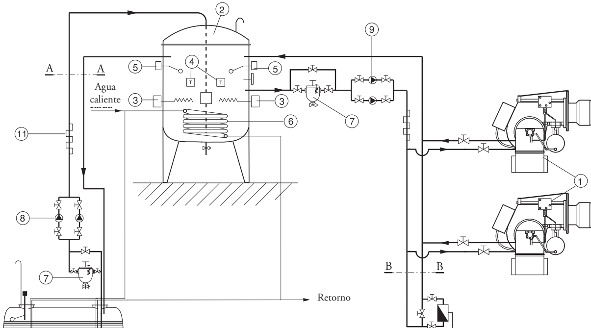
Esquema para aceite combustible fluido hasta 50°E a 50°C
