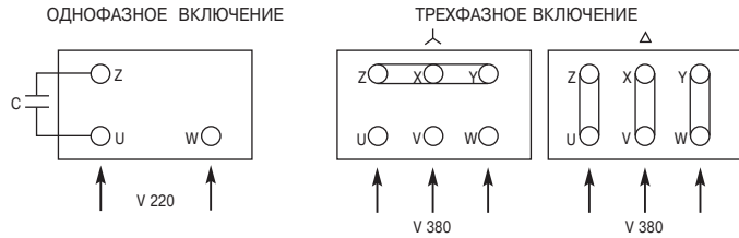
рис. 1 Подключение к электросети
