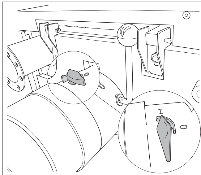
Рис. 19 Регулировка дымовой заслонки Z = ЗАКРЫТО; 0 = ОТКРЫТО
