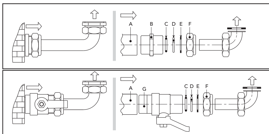
рис. 18 - Соединительный комплект
