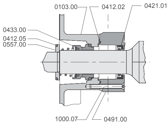
Рис. 9: Одинарное механическое уплотнение - Qiench
