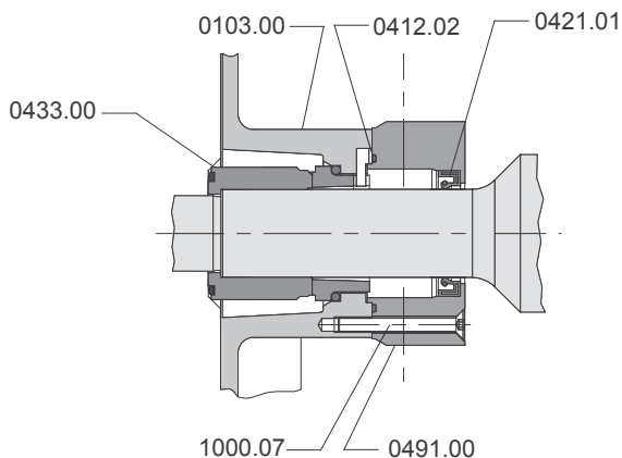
Рис. 24. Двойное охлаждаемое уплотнение – стерильное механическое уплотнение
