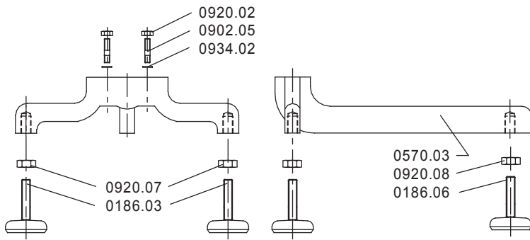
Рис. 29: Подставка BG 1
