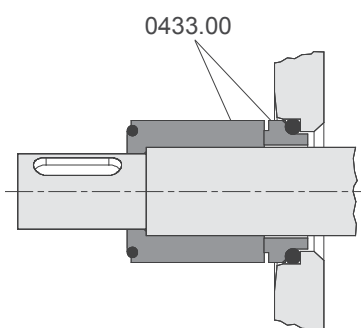
Рис. 14: Стерильное механическое уплотнение
