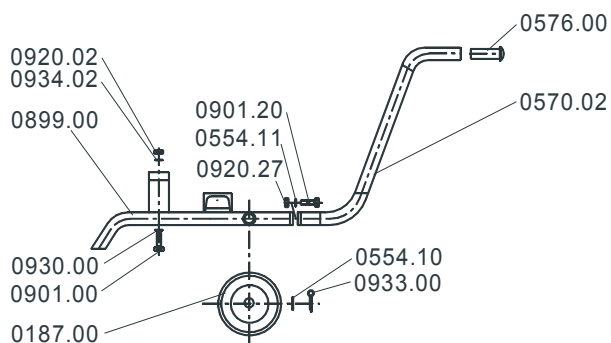
Рис. 32: Тележка.
