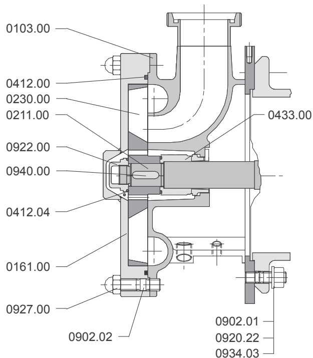
Рис. 1. Демонтаж компонентов жидкостной части
