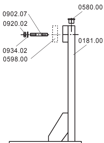
Рис. 31: Вертикальная подставка
