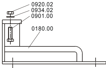
Рис. 28: Лапа VA
