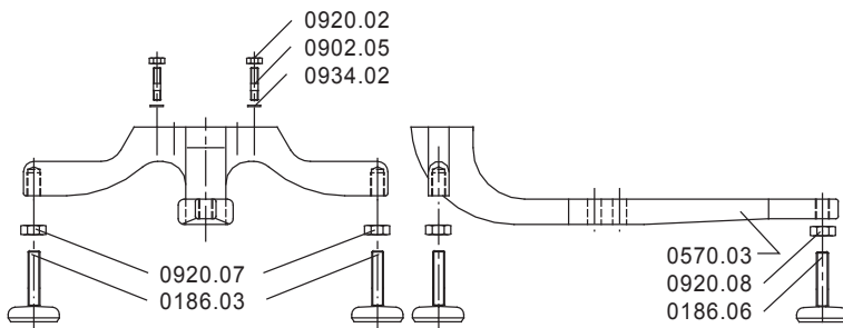
Рис. 30: Кронштейн BG 2.
