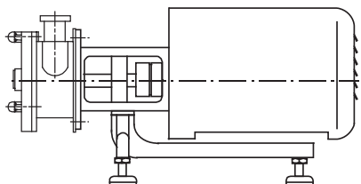
Рис. 12: SIPLA Adapta®-SUPER на шариковых опорах
