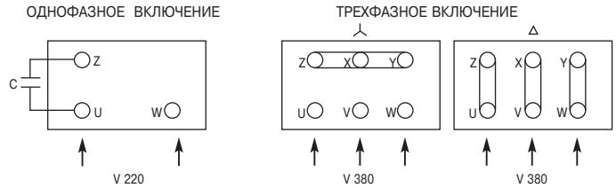
рис. 1 Подключение к электросети
