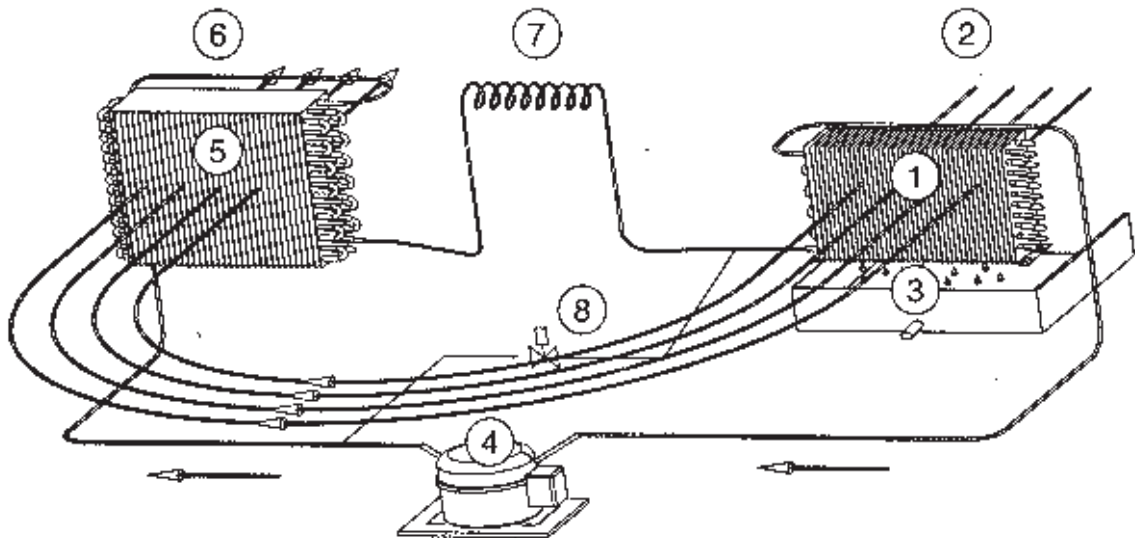
Система охлаждения
