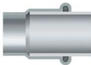
Рис. 55 Соединение в разрезе перед опрессовкой
