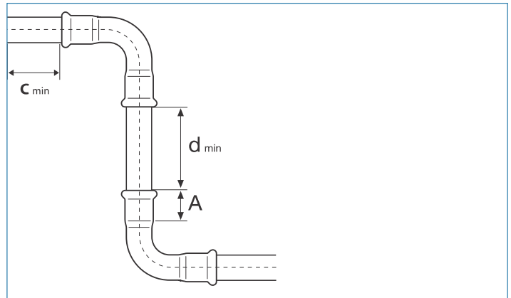
Рис. 60 Монтажные расстояния
