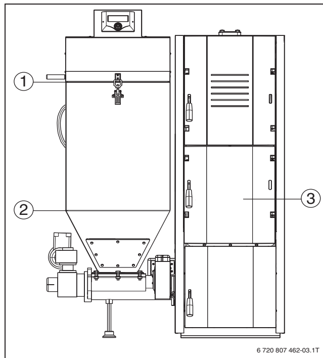
Рис. 4 Комплект поставки
