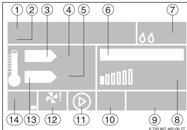
Рис. 7 Настройка отопления: рабочие параметры котла
