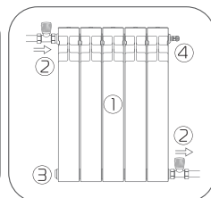
диагональное (рекомендуется для получения максимальной теплоотдачи)
