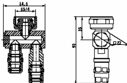
T-образное подключение системы Roth ClimaComfort
