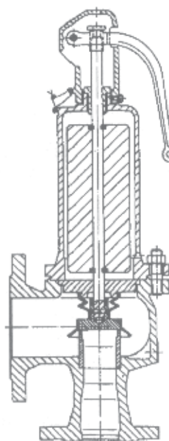
Рис. 2 Предохранительный клапан полного хода Нагрузка на вес
