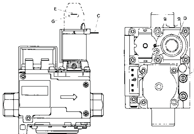
рис. 21 - Газовый клапан
