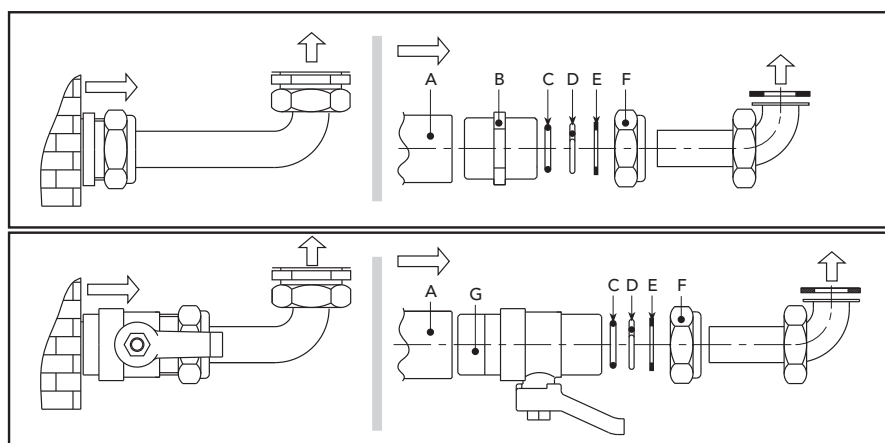
рис. 18 - Соединительный комплект
