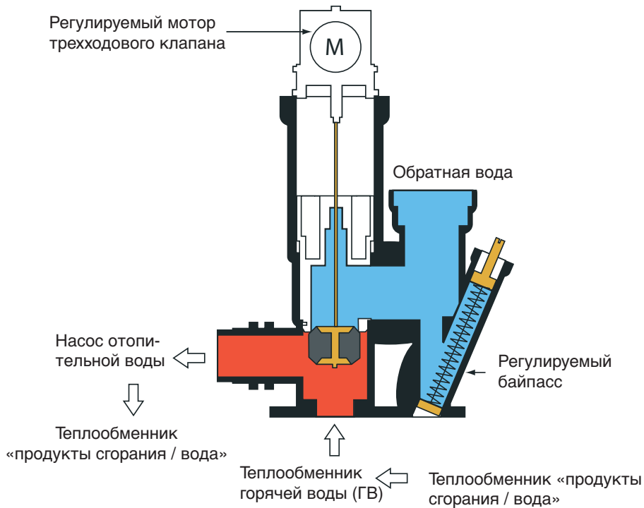
Схема работы – подготовка горячей воды (ГВ)
