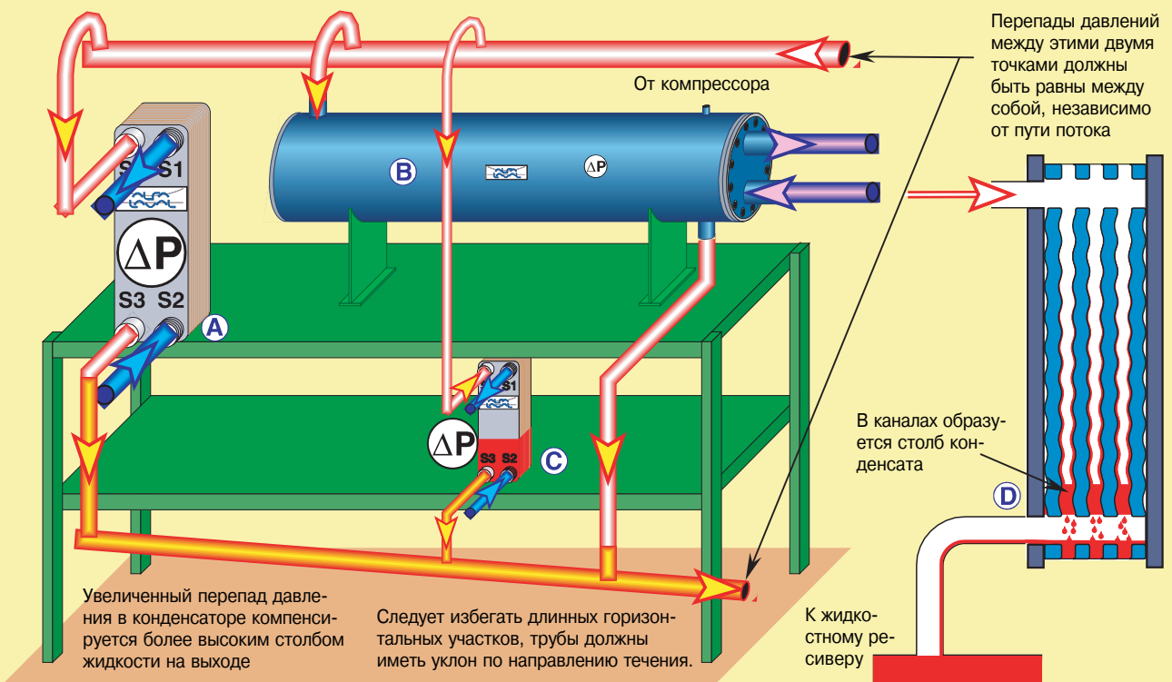
Рис. 05. Параллельно соединенные конденсаторы
