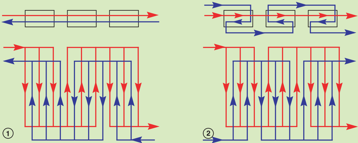
Рис. 9А. Противоток
