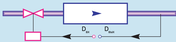
Рис. 13 Б. Разомкнутый контур ТРВ-испаритель Контур разомкнут в цепи сигнала перегрева. Изучается влияние D_{вх} на D_{вых} .
