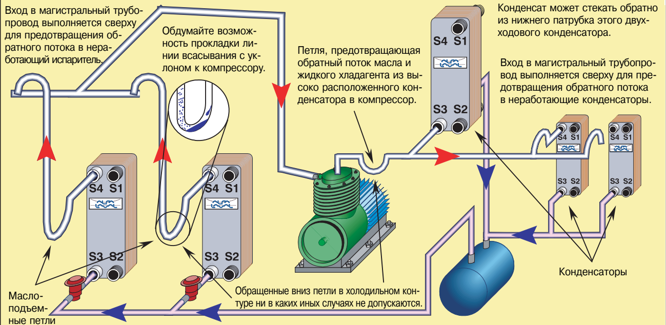
Рис. 07. Линии пара испаритель - компрессор - конденсатор
