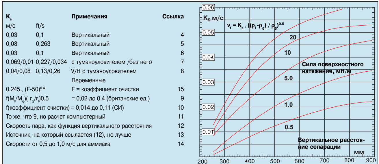
Табл. 2. Сравнение значений K_s из уравнения (4). Рис. 05. Постоянная скорости K_s
