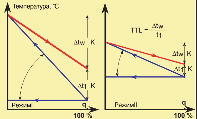
Рис. 11. Определение конечной термической длины (КТД)
