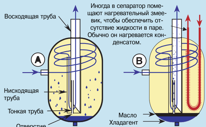
Рис. 29. Отделитель жидкости в линии всасывания
