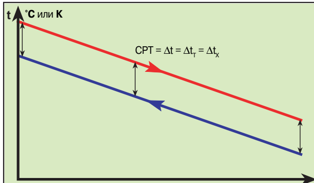
Рис. 1. Постоянная разность температур
