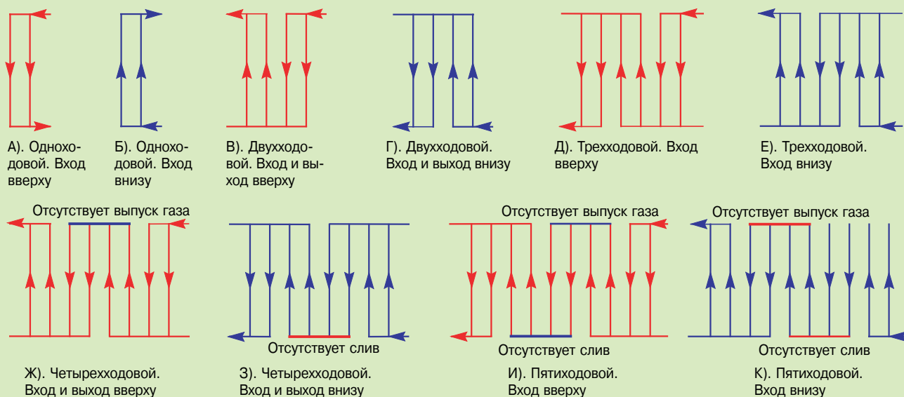
Рис. 7. Газовыпускные и сливные отверстия ППТО
