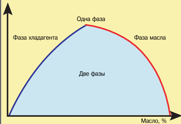
Рис. 01. Распределение масла между двумя фазами
