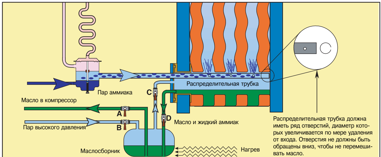
Рис. 06. Отвод нерастворимого масла из аммиачного испарителя непосредственного расширения
