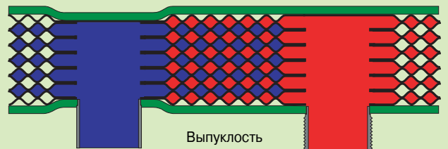
А. Конструкция с выпуклостью на задней плите.
