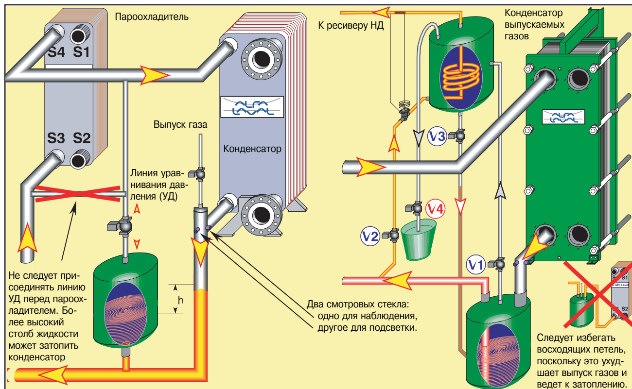
Рис. 06. Жидкостный ресивер и линия уравнивания давления
