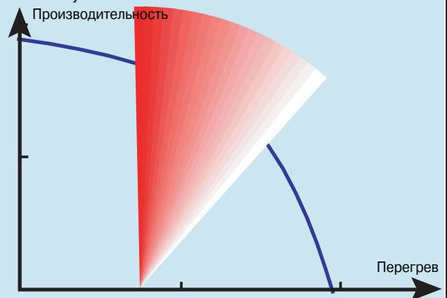
Рис. 16. Наклон кривой ТРВ
