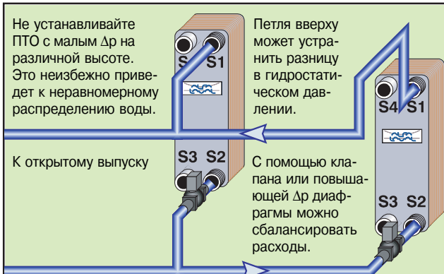
Рис. 12 А. Баланс расходов через параллельные ППТО
