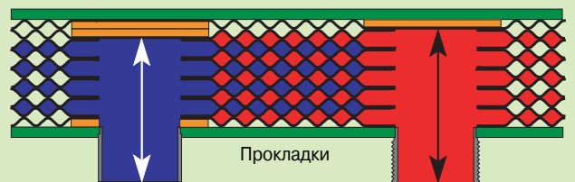
С. Теплообменник с закрытым последним каналом.
