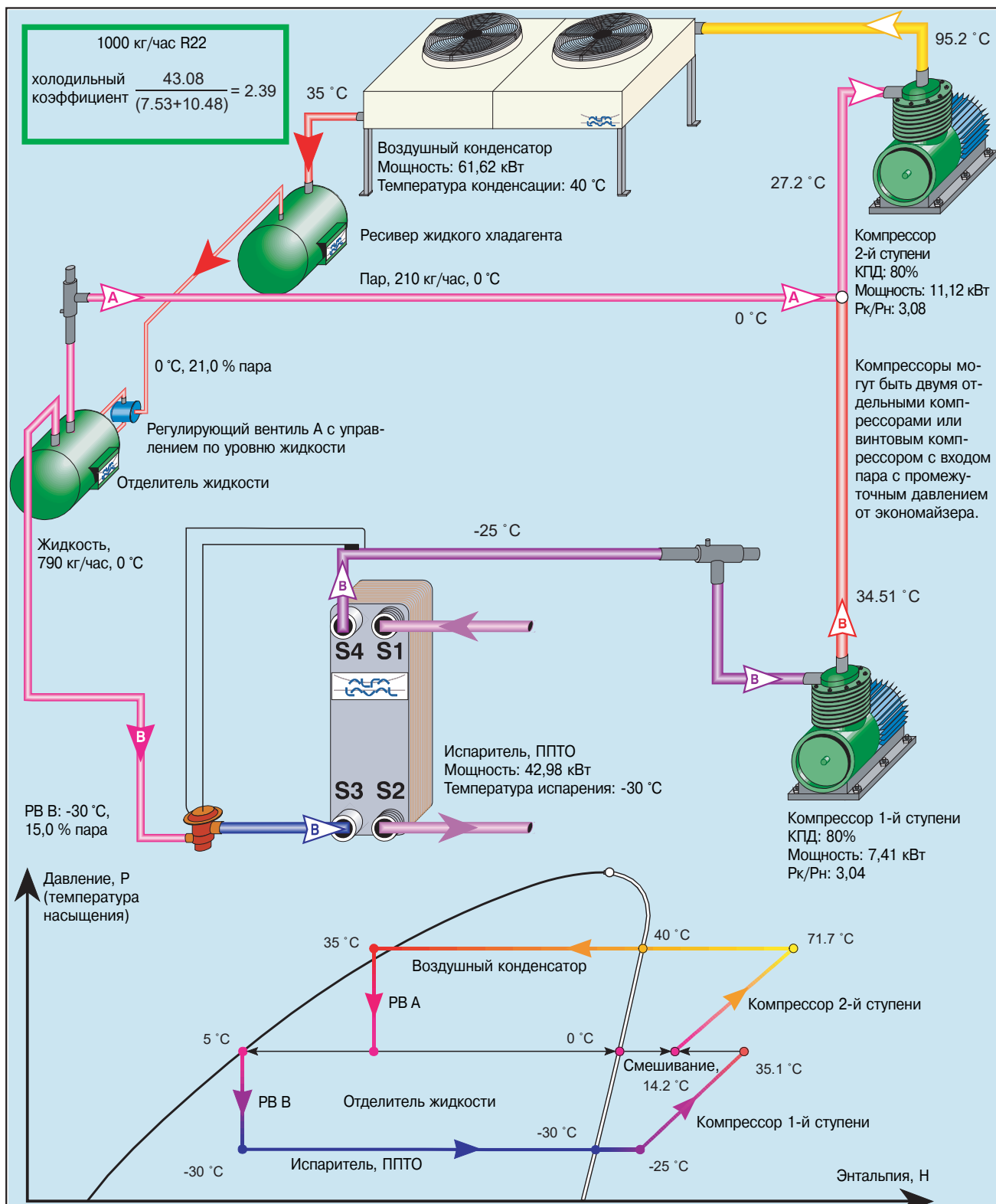
Рис. 03. Холодильный цикл с экономайзером мгновенного испарения
