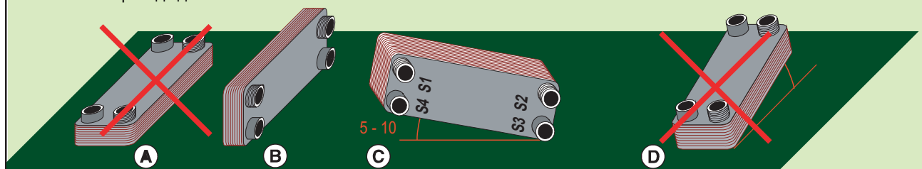
Рис. 14. Недопустимые и нежелательные положения ПТО при монтаже
