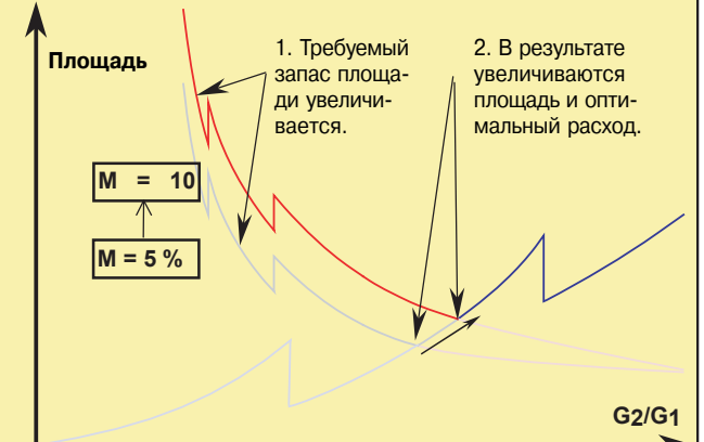
Рис. 9. Влияние увеличения запаса площади на оптимальный расход.
