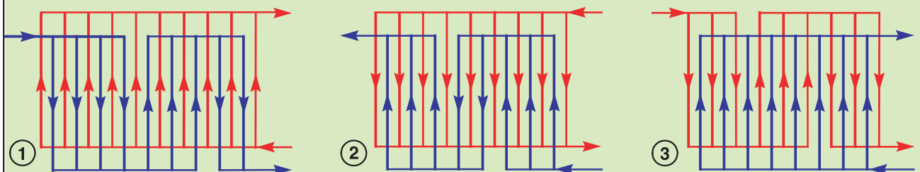
Рис. 9Б. Многоходовые схемы.
