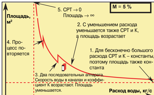
Рис. 4. Площадь как функция расхода воды при последовательном подключении ПТО.
