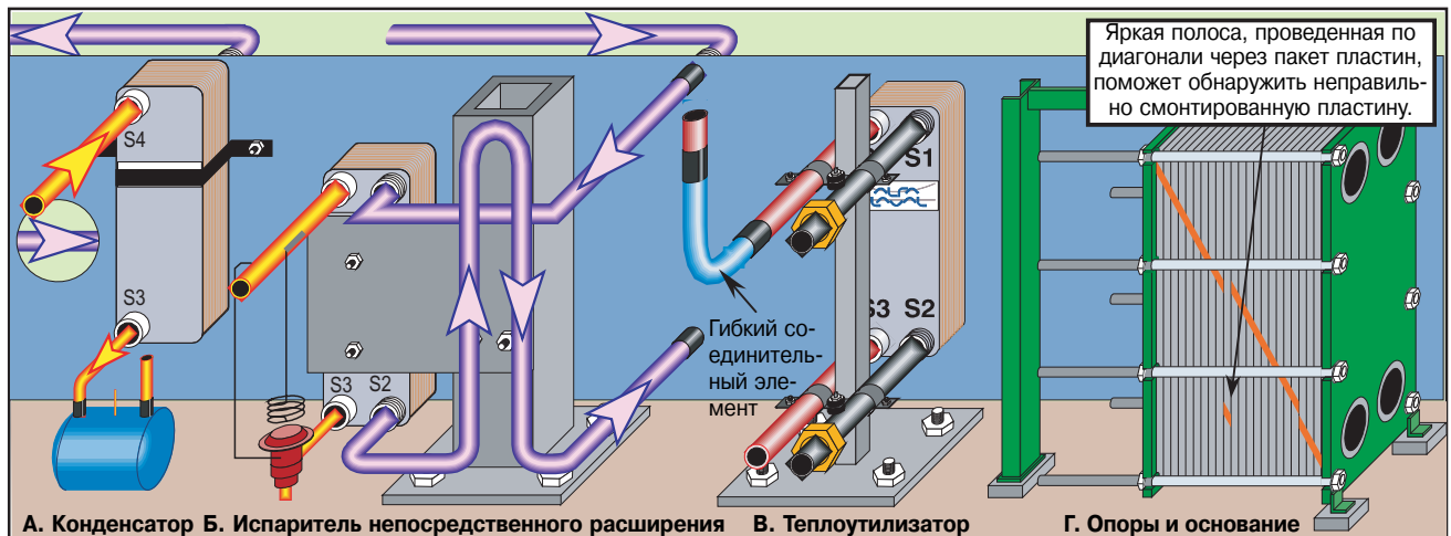
Рис. 13. Монтаж ППТО
