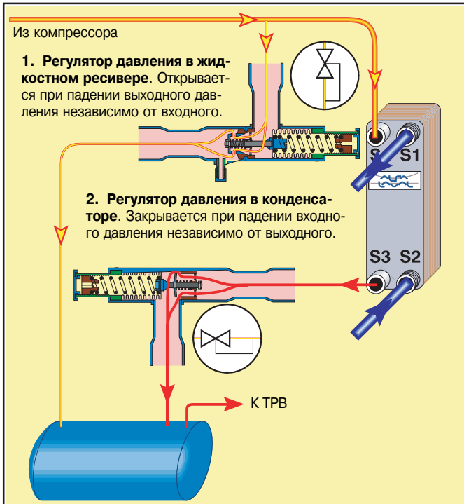
Рис. 10А. Управление давлением хладагента, способ I
