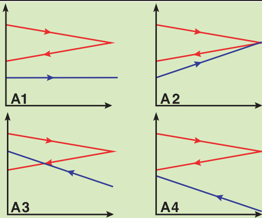
Рис. 8А. Одноходовой / двухходовой теплообменник
