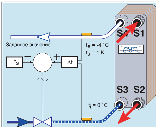
Рис. 20. Электронный регулирующий вентиль
