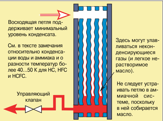
Рис. 04. Переохлаждение конденсата
