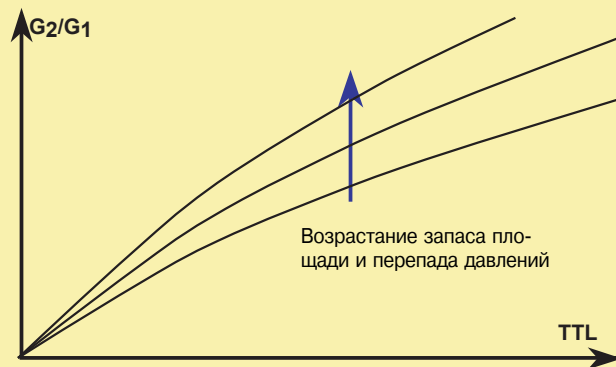
Рис. 12. Оптимальный расход как функция конечной термической длины
