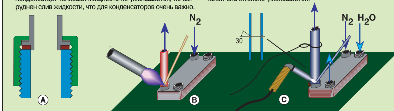
Рис. 15. Присоединение к патрубкам
