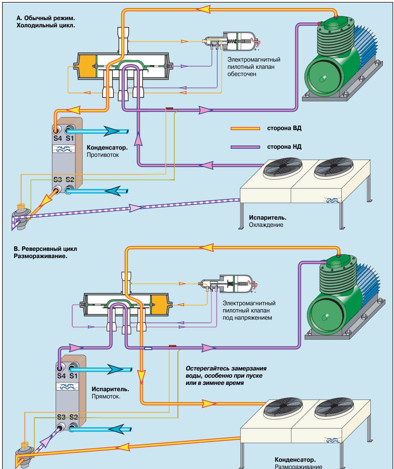
Рис. 13. Принцип действия четырехходового клапана с пилотным устройством в реверсивных холодильных установках.
