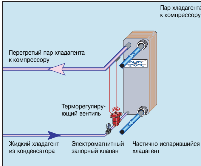
Рис. 02 А. Испаритель непосредственного охлаждения
