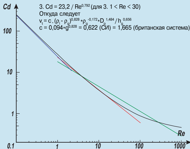
Рис. 02. Зависимость коэффициента сопротивления C_d от Re
