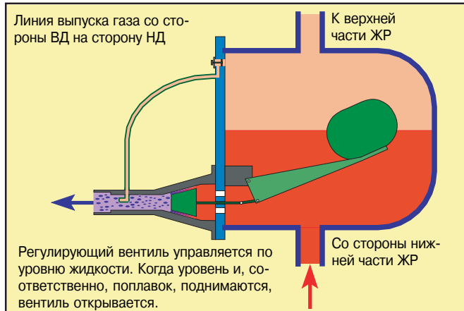
Рис. 07. Регулирующий клапан с управлением по уровню жидкости и отводом газов из ресивера ВД
