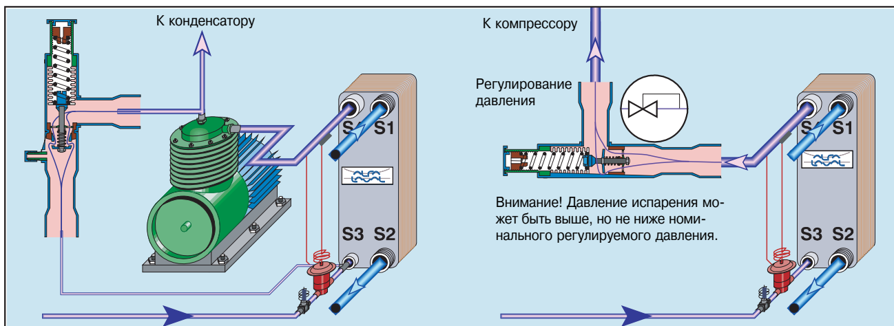
Рис. 23. Регулятор испарителя непосредственного расширения с перепуском горячего пара
