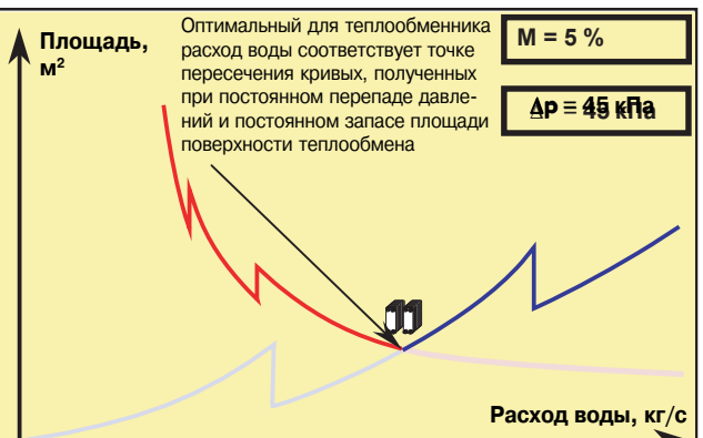
Рис. 5. Тепловые и гидравлические характеристики соответствуют требованиям
