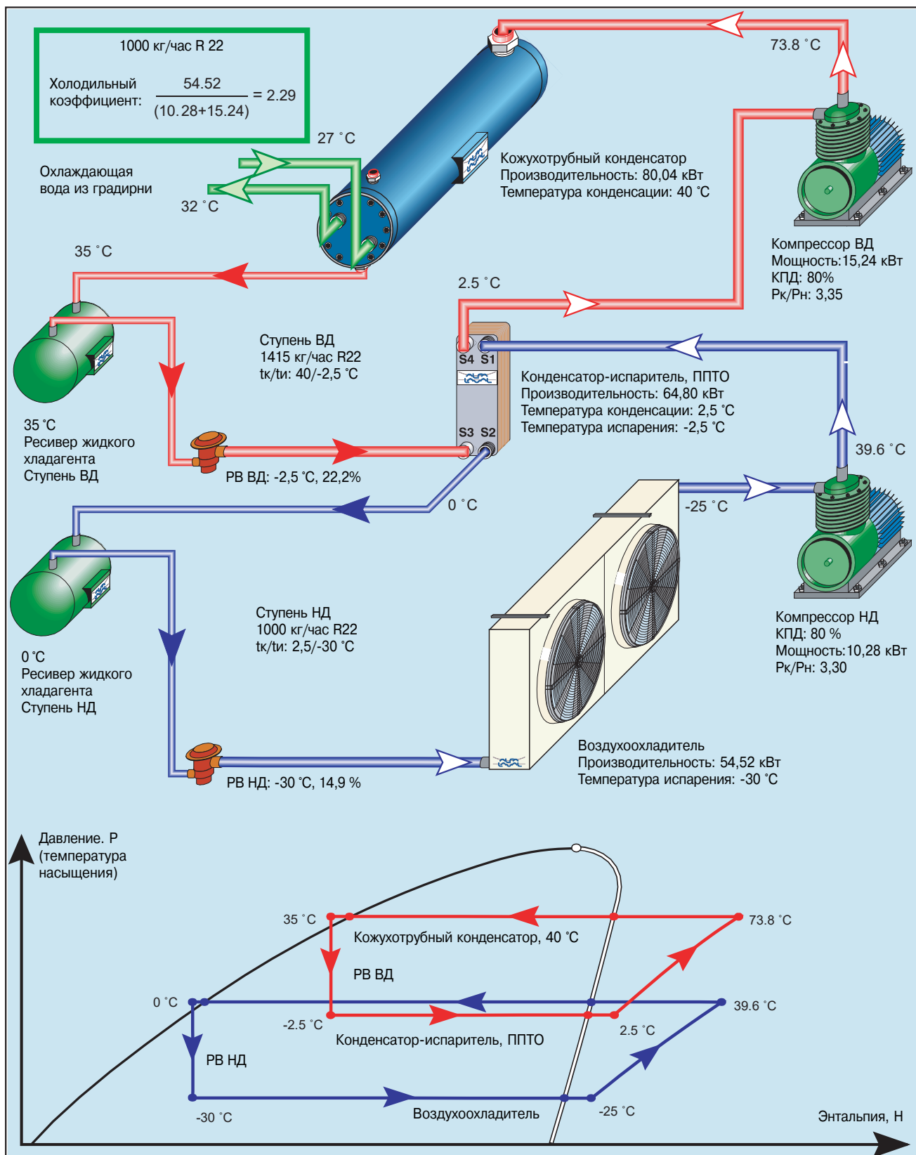
Рис. 06. Каскадный холодильный цикл
