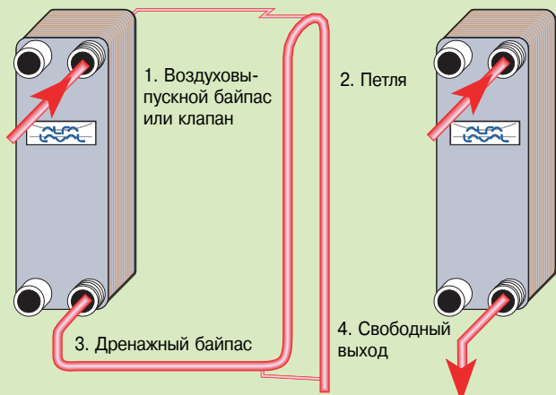
Рис. 12 Б. Верхняя петля с байпасом
