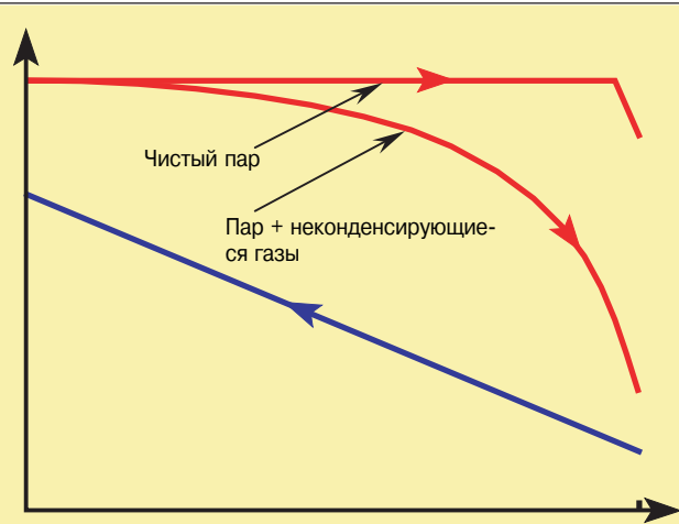
Рис. 03. Пар с неконденсирующимися газами
