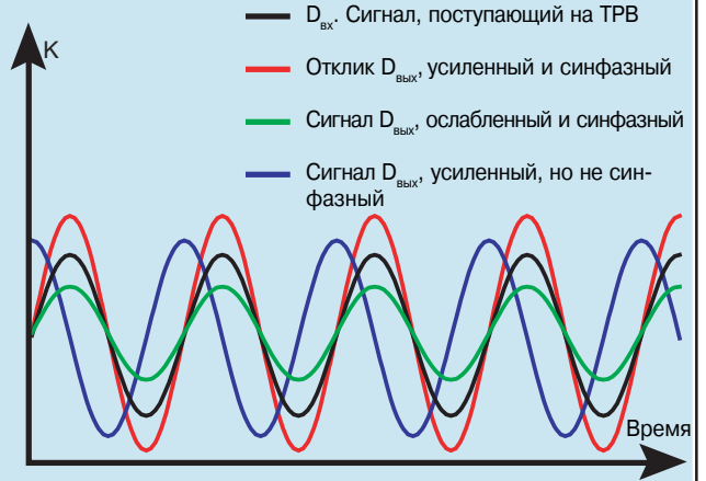
Рис. 13 В. Динамическая характеристика На рисунке показаны возможные отклики D_{вых} при синусоидальном сигнале D_{вх} .
