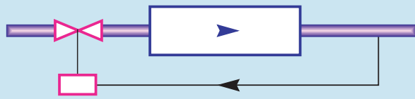
Рис. 13 А. Контур ТРВ-испаритель Испаритель и ТРВ образуют замкнутый контур, в котором перегрев является входным сигналом для ТРВ.
