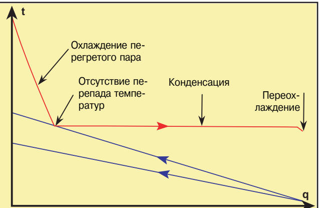
Рис. 18. Режимы конденсатора с различными расходами воды
