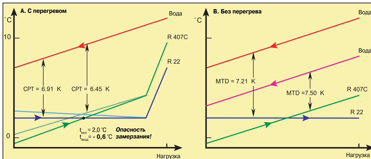
Рис. 13. CPT для R22 и R407C
