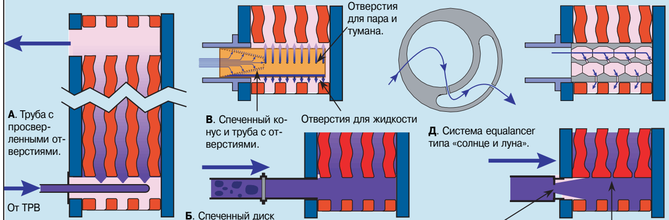
Рис. 18. Распределитель хладагента
