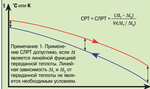
Рис. 3. Нелинейное изменение разности температур
