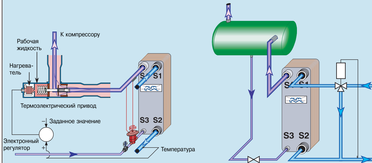
Рис. 25. Электронный регулятор давления испарения
