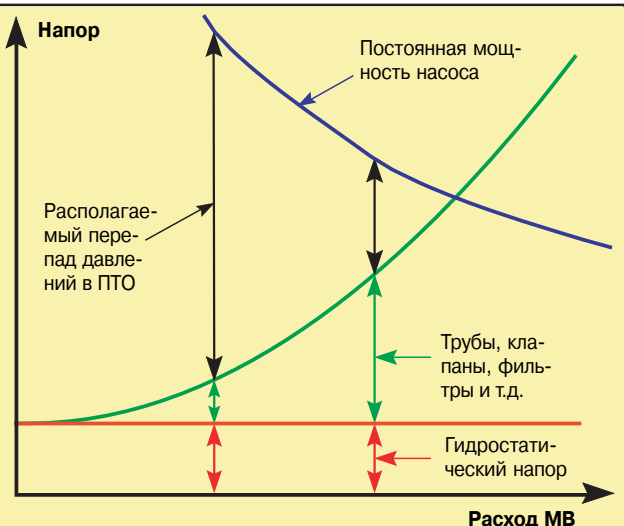
Рис. 22. Распределение перепада давлений
