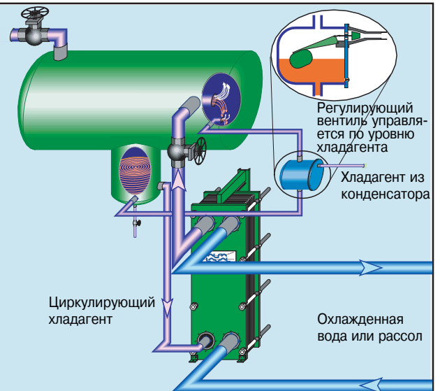
Рис. 02 Б. Термосифонный испаритель
