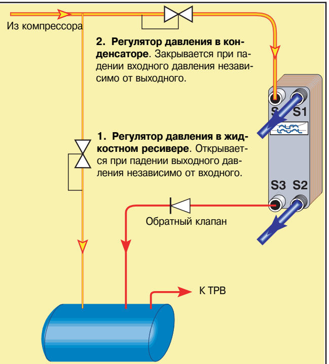
Рис. 10В. Управление давлением хладагента, способ II
