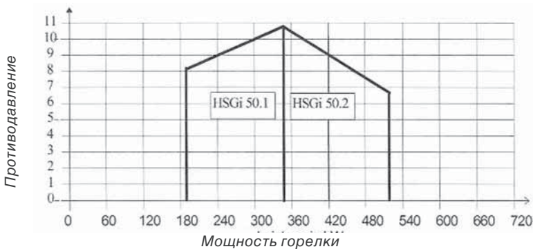
Рис.39 Рабочее поле горелки
