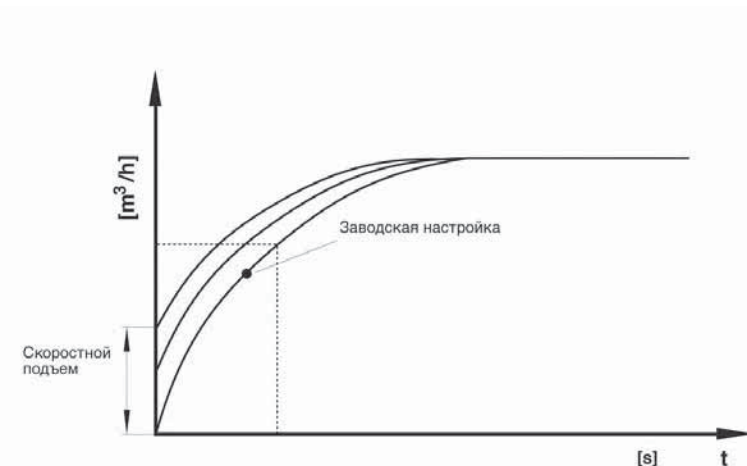
Рис.19 Настройка скоростного подъема
