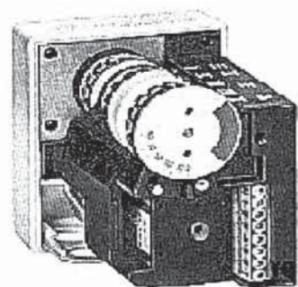
Рис.37 Сервомотор SQN 31.151 HSGi 22/ 50.1
