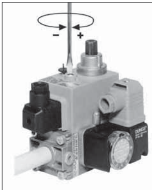
Рис.13 Регулировка динамического давления MB- DLE ... B01
