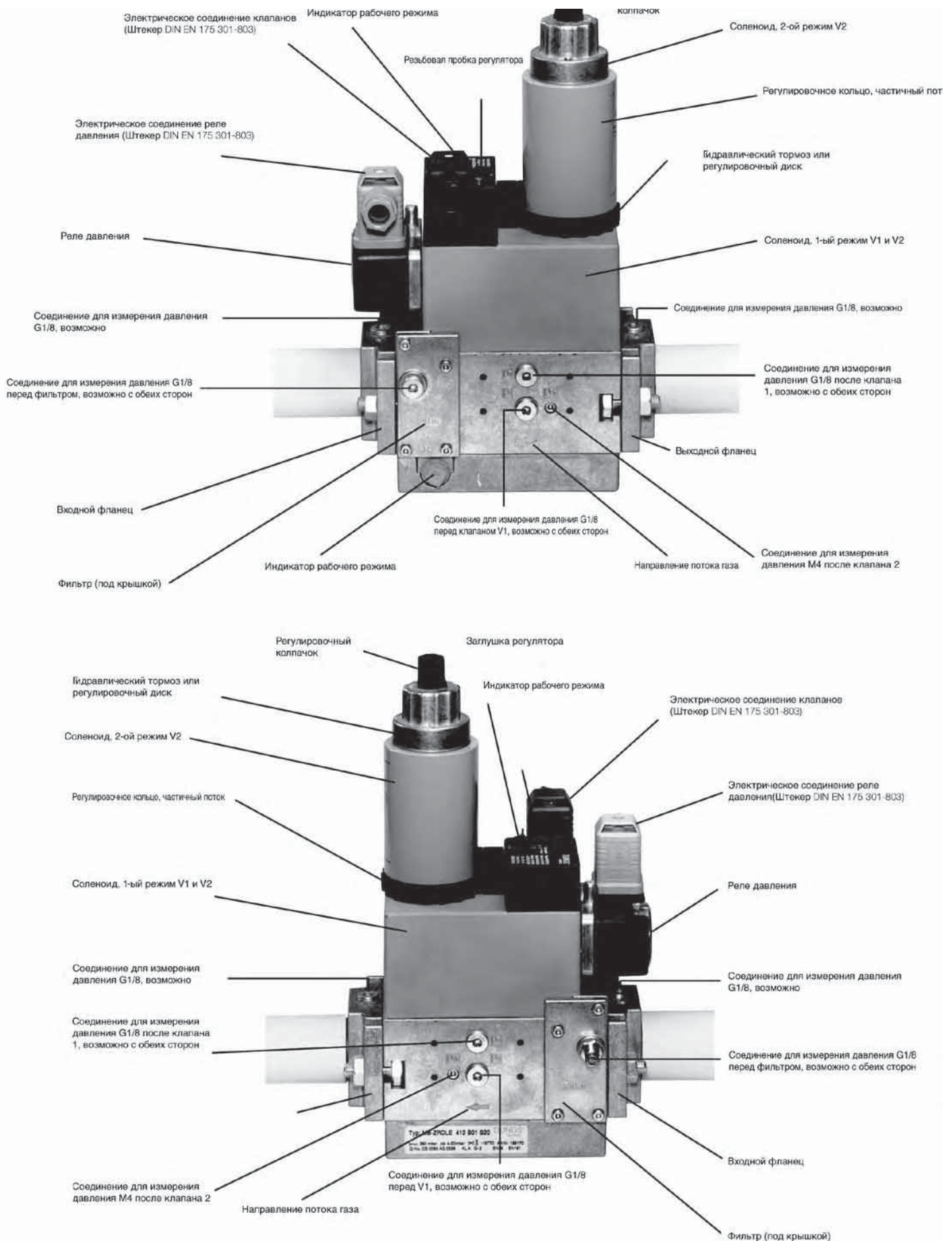
Рис. 11 Газовый МультиБлок MB ZR DLE ...B01HSGi 12.xZ, HSGi 22 Z, HSGi 50.1Z
