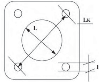
Рис.1 Соединительный фланец
