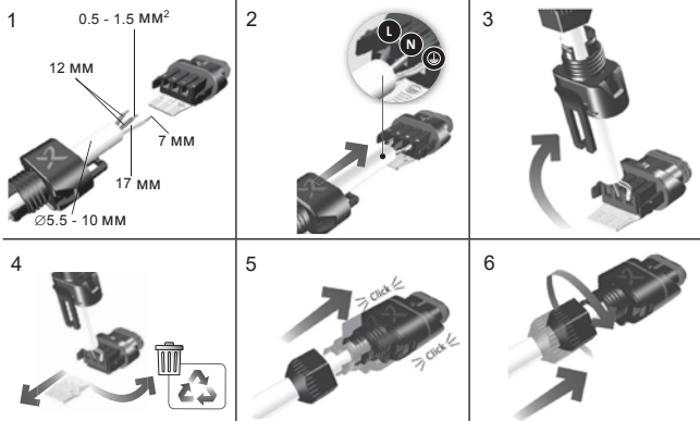
9-сүр. Электр туташтыргычы орнотуу
