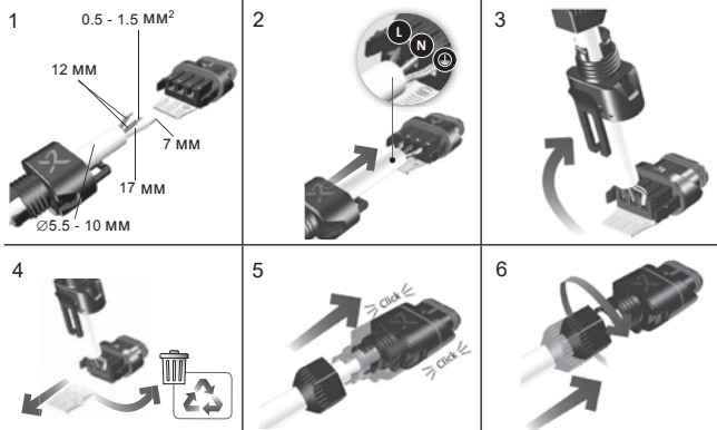
Рис. 9 Установка электроразъема
