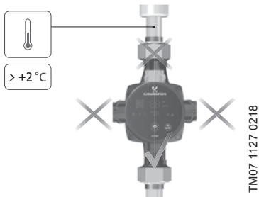
Նկար 6 Կառավարման բլոկի դիրքն օդորակման և ՍՋ համակարգերում պոմպի տեղադրման ժամանակ
