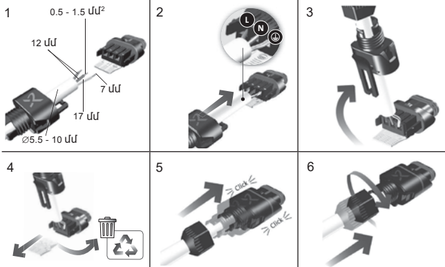
Նկար 9 Էլեկտրական հարակցիչի տեղադրումը
