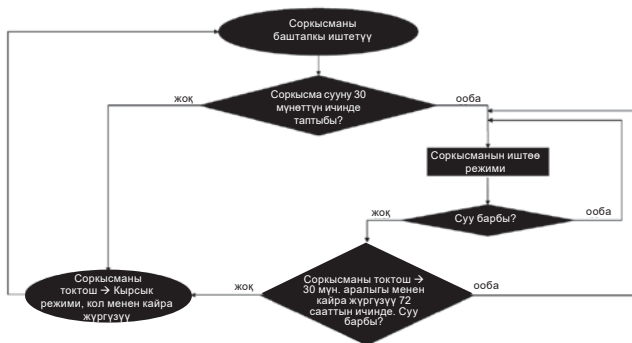
25-сүр. «Куру» иштөөдөн коргоонун иштөө алгоритми
