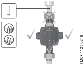
Նկար 5 Կառավարման բլոկի դիրքը ջեռուցման և SՋ տեղական համակարգերում պոմպի տեղադրման ժամանակ
