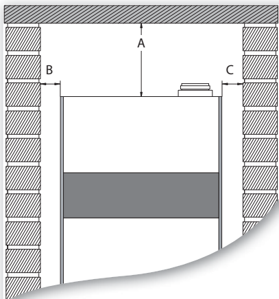
Вид спереди
