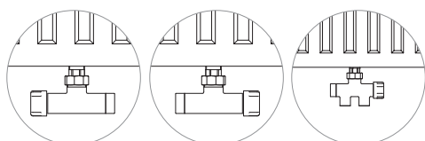
Клапан с погружающей трубкой угловой левой
