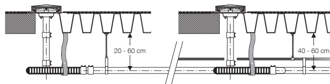
Рис. 89: Монтаж соединительной трубки flexibles до высоты свешивания ≤ 0,6 м
