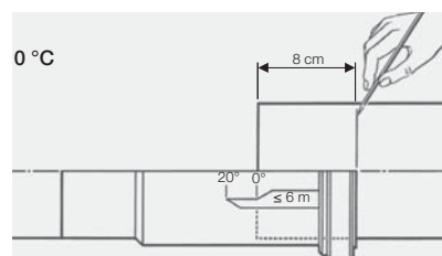
Рис. 84: Глубина вставки при температуре монтажа 0 °C
