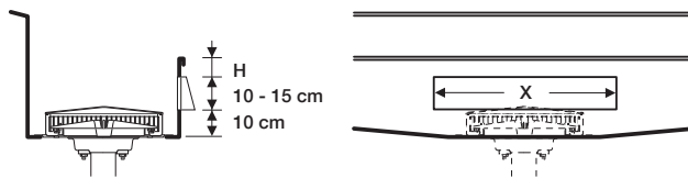
Рис. 68: Аварийный перелив в желобе, в продольной стороне
