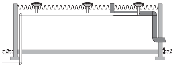
Рис. 73: Система Pluvia с аварийным отводом воды через традиционную трубопроводную систему
