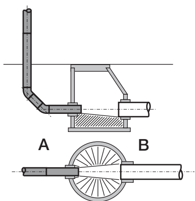
Рис. 52: Расширение путем выпуска в смотровой колодец
