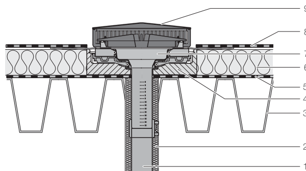
Рис. 34: Конструкция легкой кровли, изолированной, с кровельным покрытием
