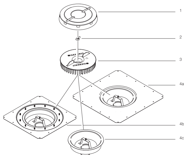
Рис. 10: Компоненты воронок Pluvia объемом 25 л
