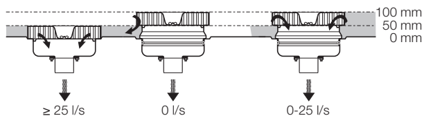
Рис. 15: Принцип действия аварийного перелива Pluvia 25 л
