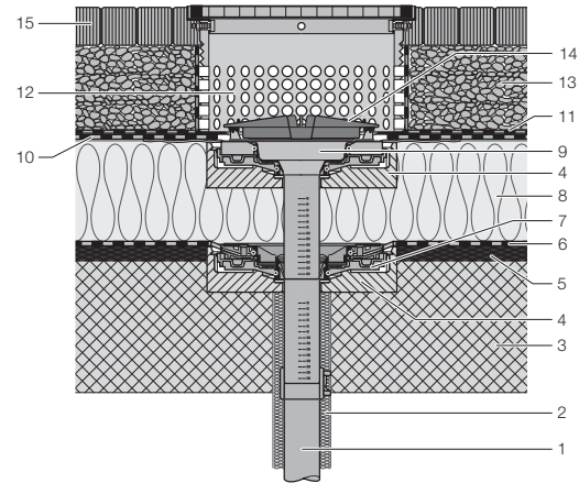
Рис. 31: Конструкция монолитной крыши, с пароизоляцией и кровельным покрытием, пригодным для передвижения людей
