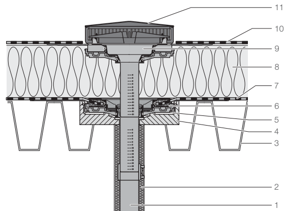
Рис. 36: Конструкция легкой кровли, изолированной, с креплением пароизоляции
