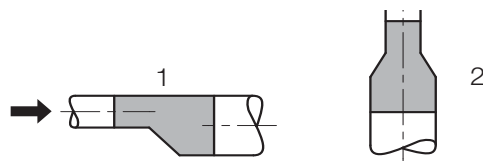
Рис. 48: Эксцентрические и концентрические переходы
