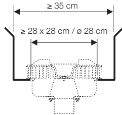
Рис. 80: Легкая кровля
