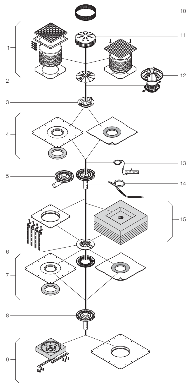
Рис. 7: Обзор всех применяемых компонентов воронок Pluvia модульной конструкции для отвода дождевой воды с крыши объемом 12 л
