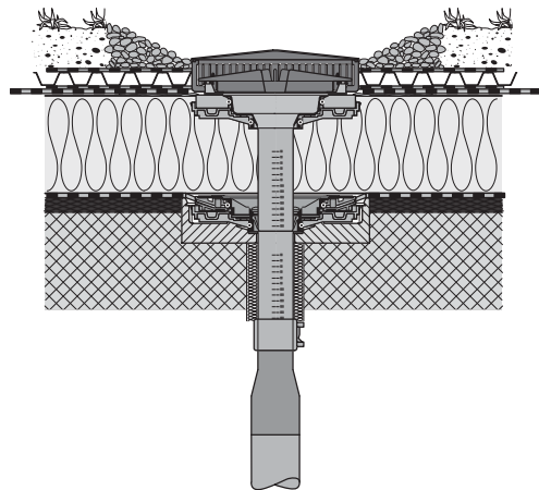
Рис. 47: Подсоединение воронки Pluvia с помощью расширяющегося переходника
