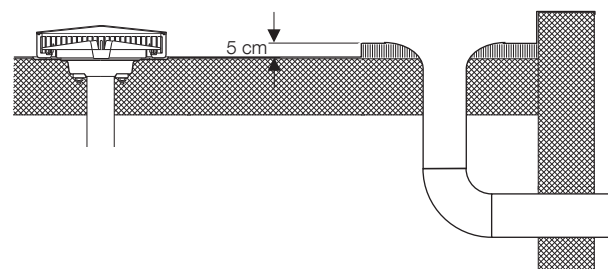
Рис. 74: Традиционный аварийный отвод воды как конструктивная мера
