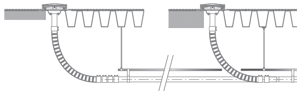
Рис. 88: Монтаж соединительной трубки flexibles с высотой свешивания > 0,6 м
