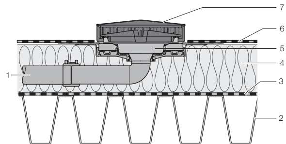
Рис. 37: Конструкция легкой кровли, изолированной, горизонтальный излив в тепловой изоляции, с кровельным покрытием и пароизоляцией
