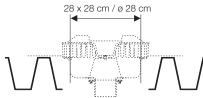
Рис. 80: Легкая кровля
