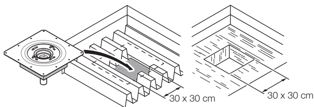
Рис. 78: Монолитная кровля
