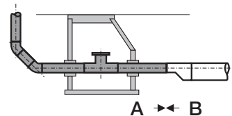
Рис. 53: Расширение после смотрового колодца, допускаемое
