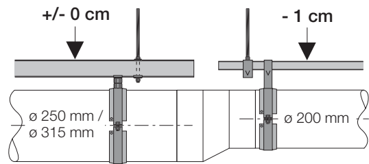
Рис. 63: Не соединяемые несущие шины
