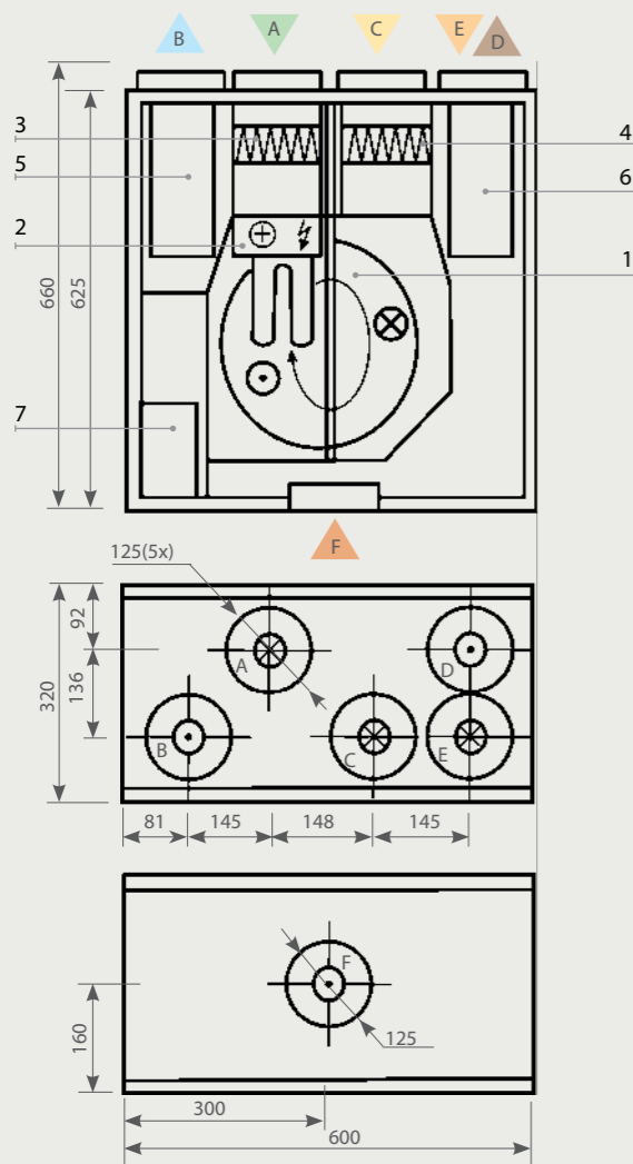
REGO 200V Левая сторона
