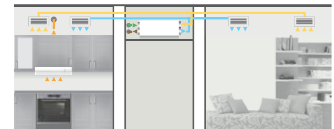
Сбалансированная система вентиляции в помещениях
