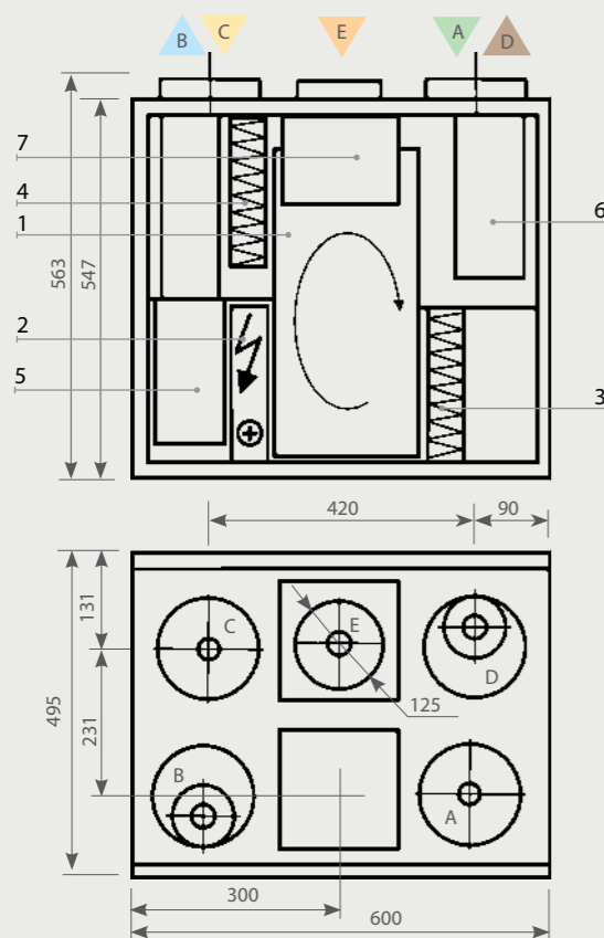
REGO 400V Левая сторона
