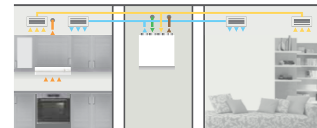
Сбалансированная система вентиляции помещений
