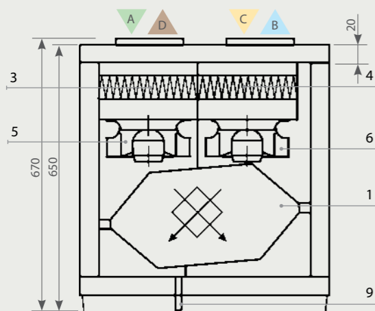
RECU 400V CF Правая сторона
