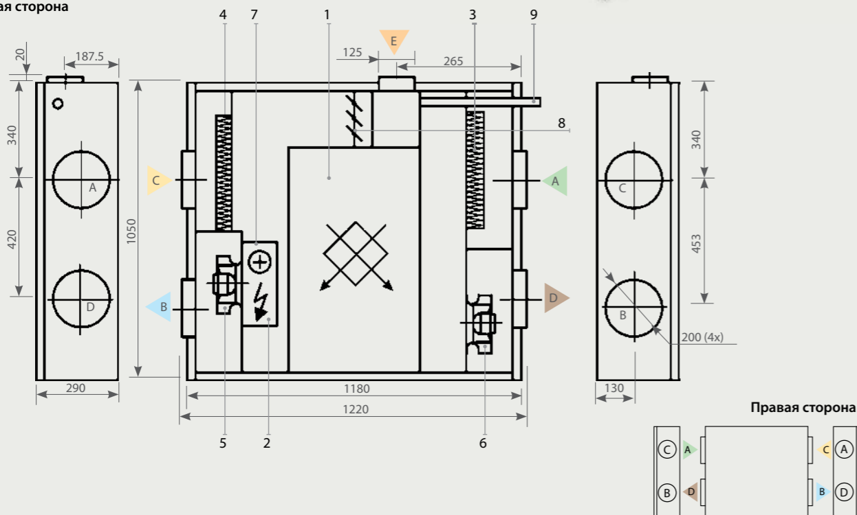
RECUC 500P CF Левая сторона
