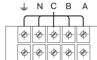
Рис. 3. Схема подключения
