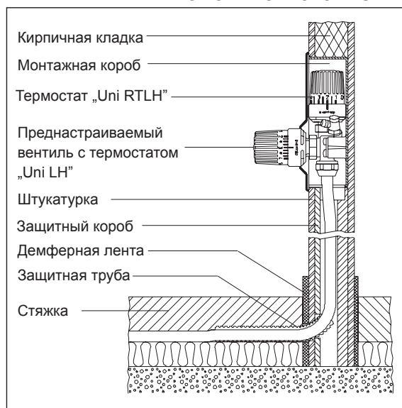
„Unibox plus”, строительная глубина 57 мм
