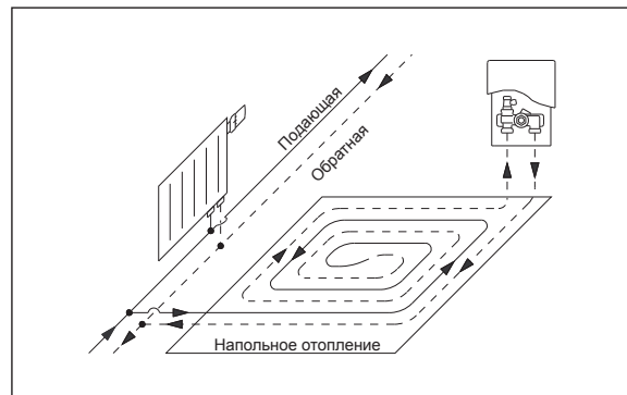
Схема монтажа: ограничение т-ры обратного потока
