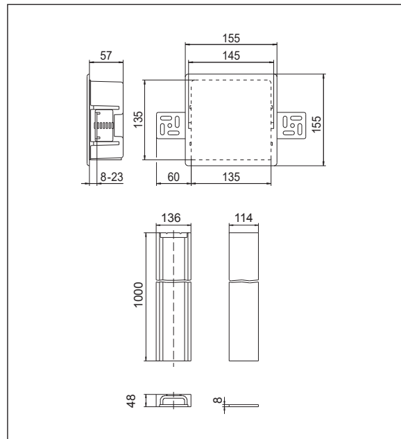
Размеры „Unibox E RTL” и защитного короба
