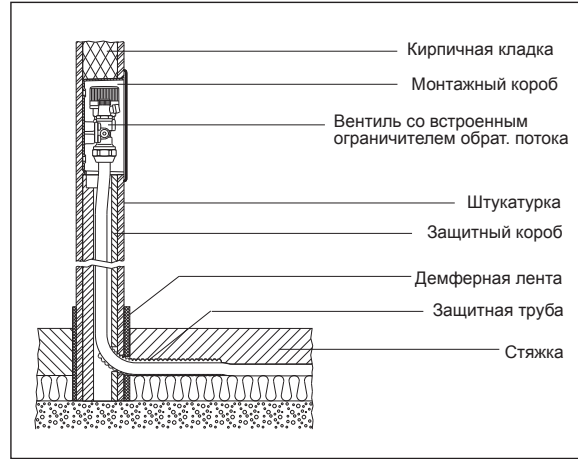
„Unibox E RTL”, строительная глубина 57 мм
