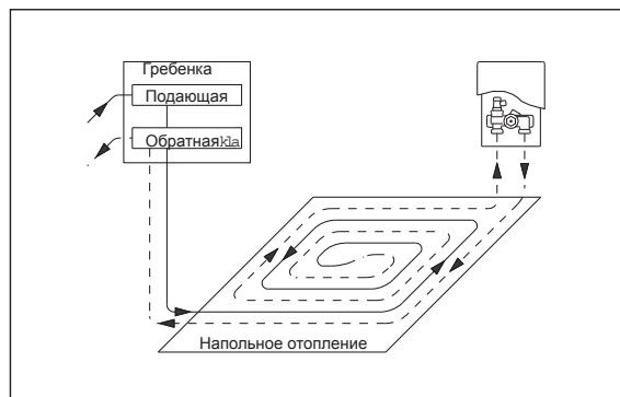
Схема монтажа: регулирование т-ры отдельного помещения
