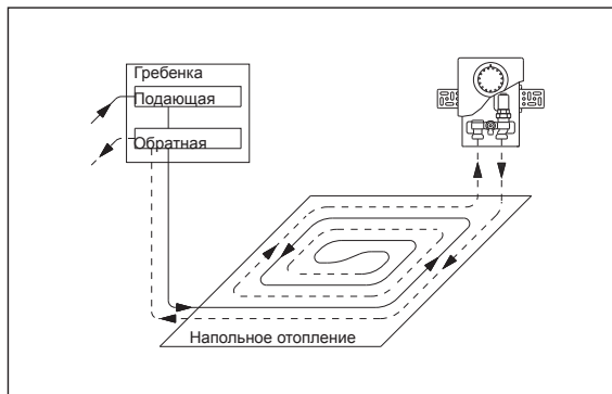
Схема монтажа: регулирование температуры отдельного помещения
