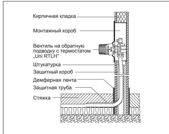
„Unibox RTL”, строительная глубина 57 мм
