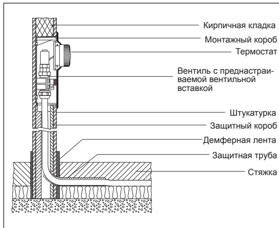
„Unibox E T”, строительная глубина 57 мм
