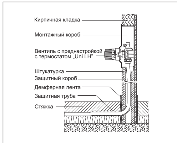
„Un box T”, строительная глубина 57 мм
