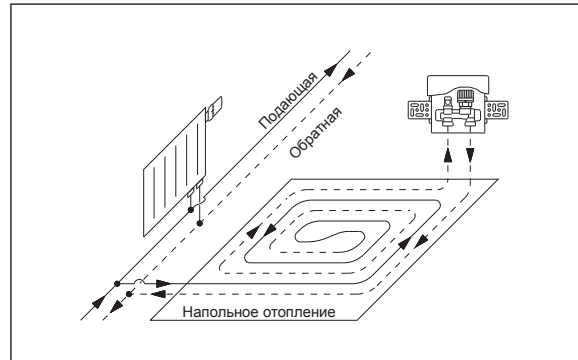
Схема монтажа: ограничение температуры обратного потока
