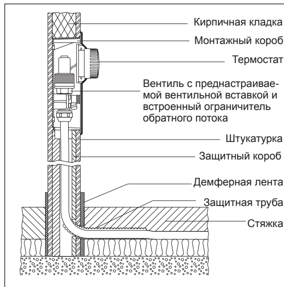
„Unibox E plus”, строительная глубина 57 мм
