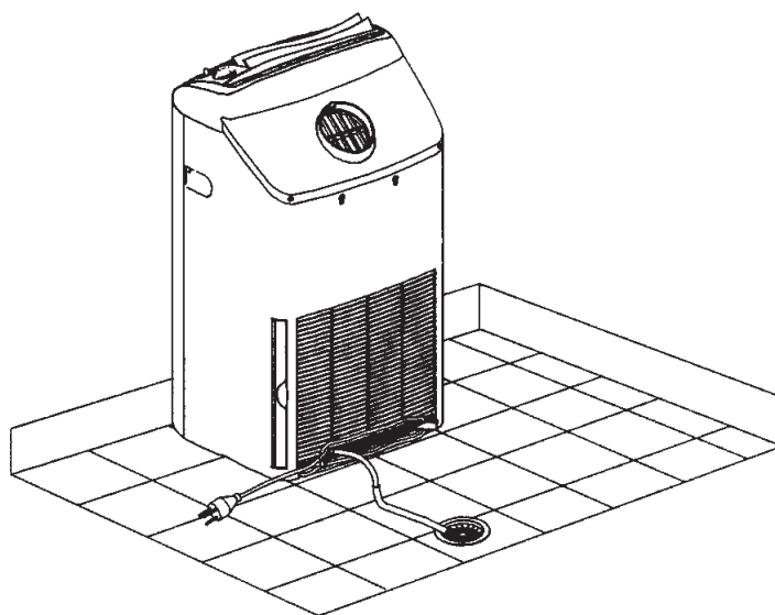
Рис. 8. Монтаж кондиционера, работающего в режиме влагуудаления
