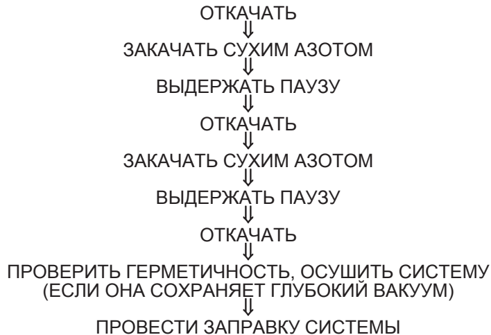
Рис. 8 — Метод тройной откачки
