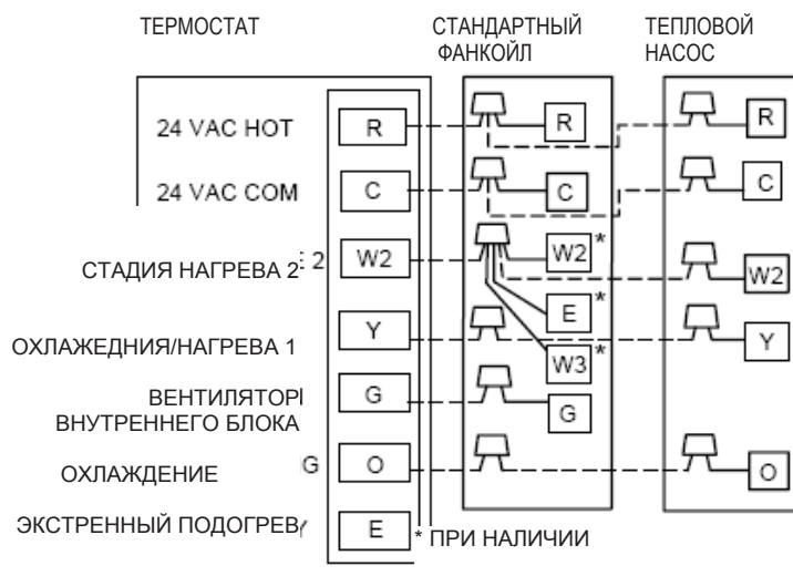
Рис. 10 Типовая электрическая схема (См. инструкции по установке термостата – там даны комбинации подключений к агрегату)
