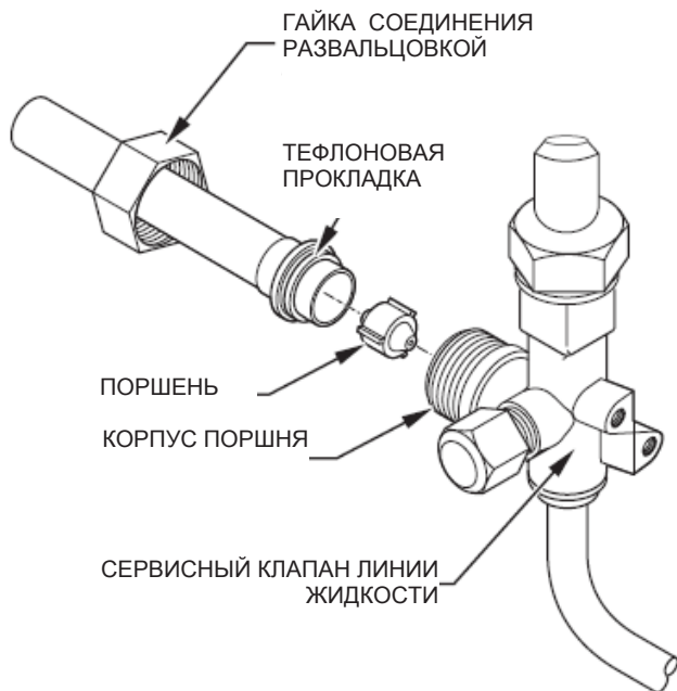
Рис. 5—Сервисный клапан линии жидкости с переходной трубкой
