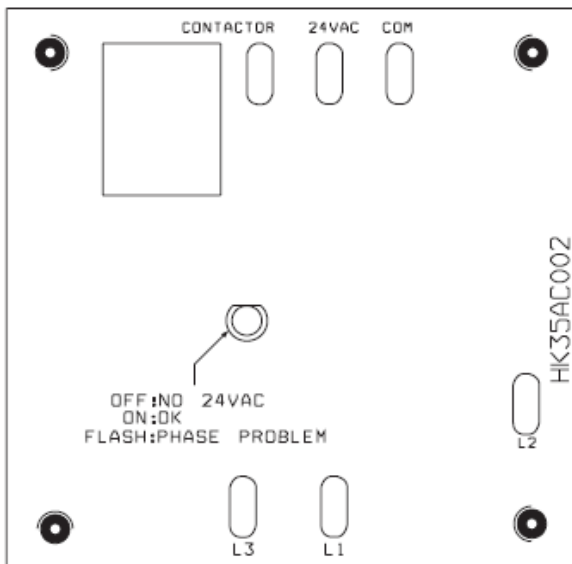
Рис. 11 Монитор фаз
