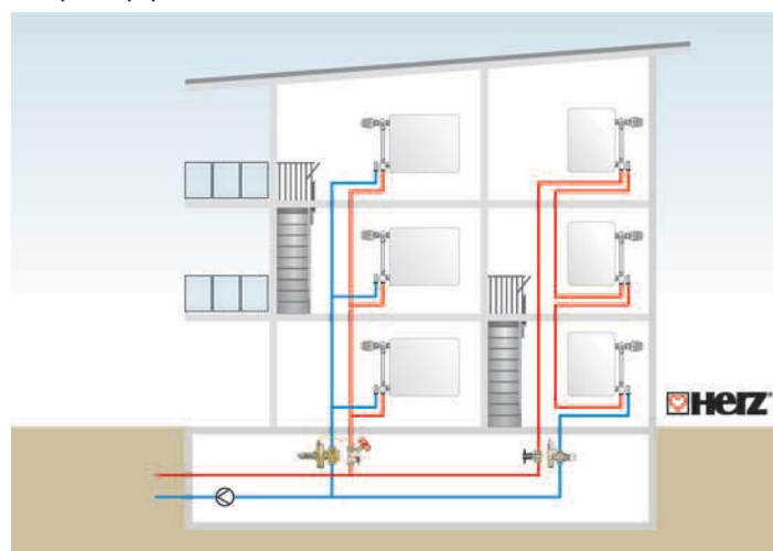
Слева - двухтрубная система отопления с регулятором перепада давления
