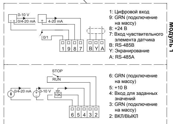
Рис. 4 Схема соединений – TPE
