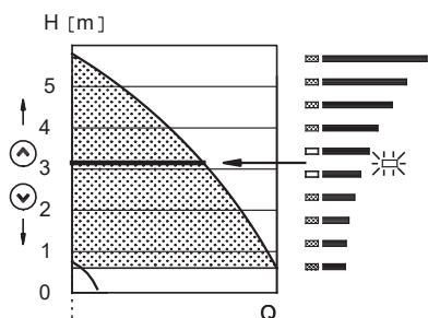
Рис. 17 Насос с регулированием постоянного давления
