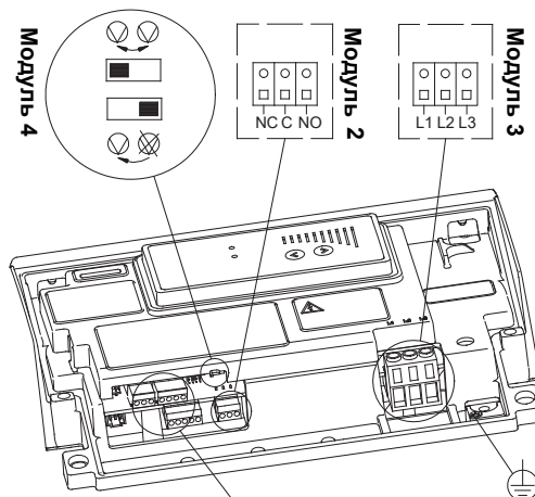
Рис. 4 Схема соединений – TPE
