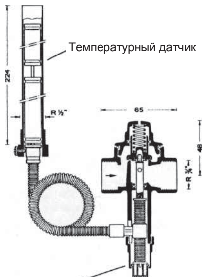
Сильфонная система
