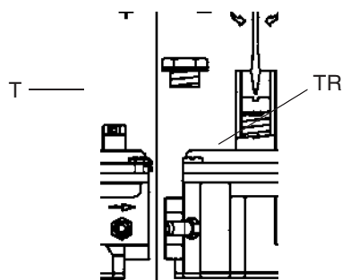
Стабилизатор давления
