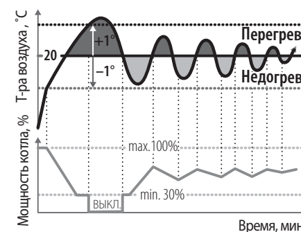
Работа пропорционального (модулирующего) комнатного термостата при поддержании 20°C
