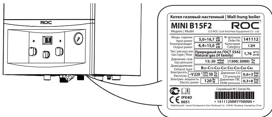
Пример шильдика котла
