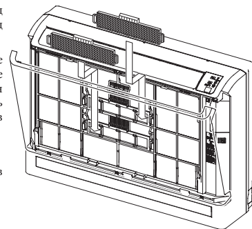
Оправка фильтра
