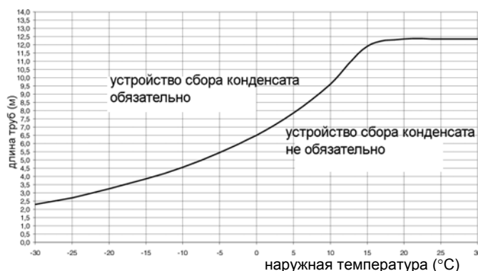
Коаксиальные дымоотвод/воздуховод
