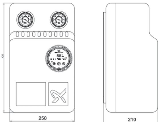
Рис. 45 Габаритные размеры
