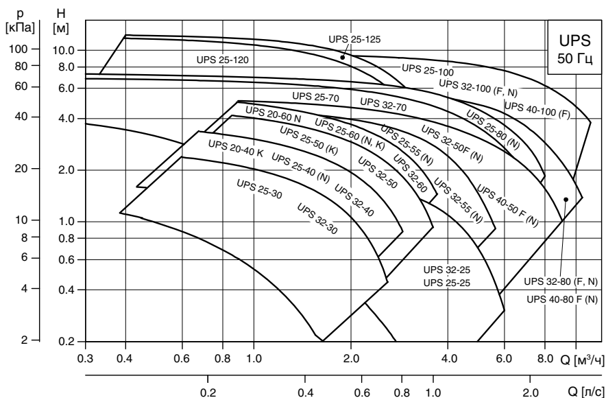
Рис. 25 Расходно-напорная характеристика насосов UPS
