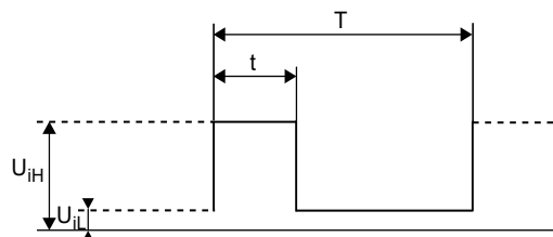
Рис. 69 ШИМ-сигнал
