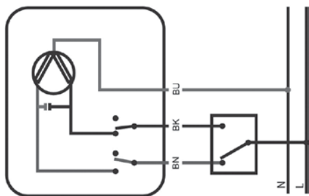
Рис. 52 Электрическая схема
