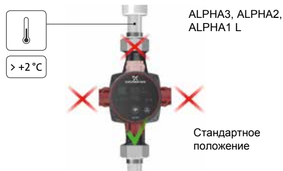
Рис. 17 Возможное положение блока управления для системы отопления
