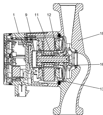
Рис. 14 Насос ALPHA3/ALPHA2/ALPHA1 L
