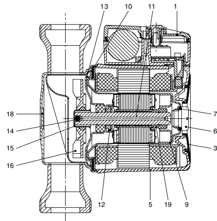
Рис. 33 Однофазный насос UP
