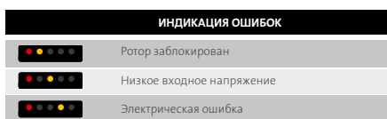
Рис. 71 Индикация ошибок
