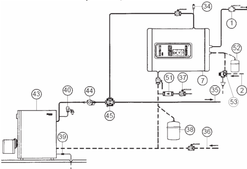
Автономный котел с трехпозиционным клапаном
