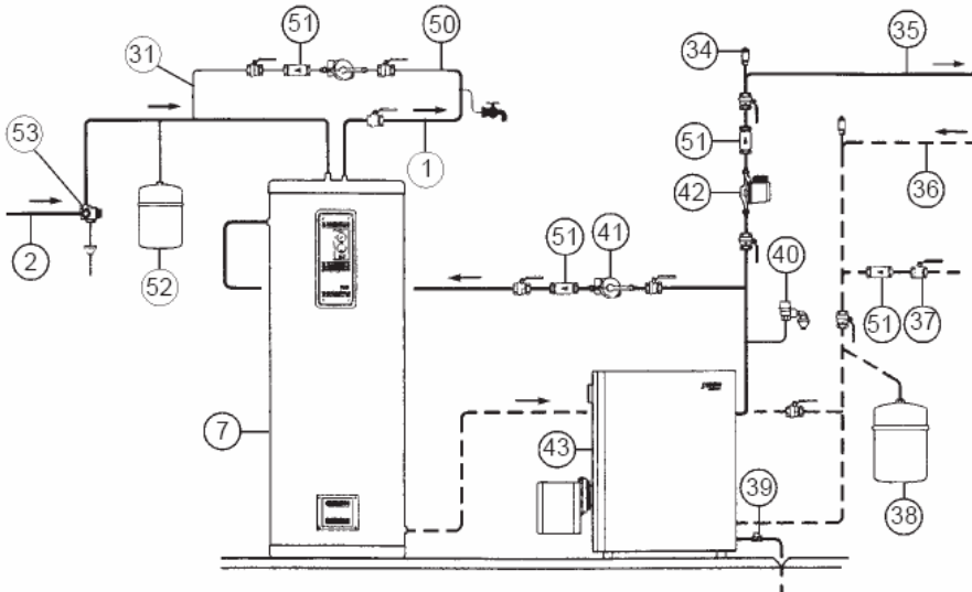
Автономный котел с трехпозиционным клапаном
