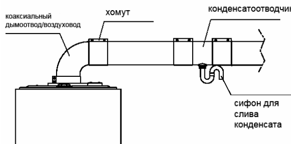
Коаксиальные дымоотвод/воздуховод
