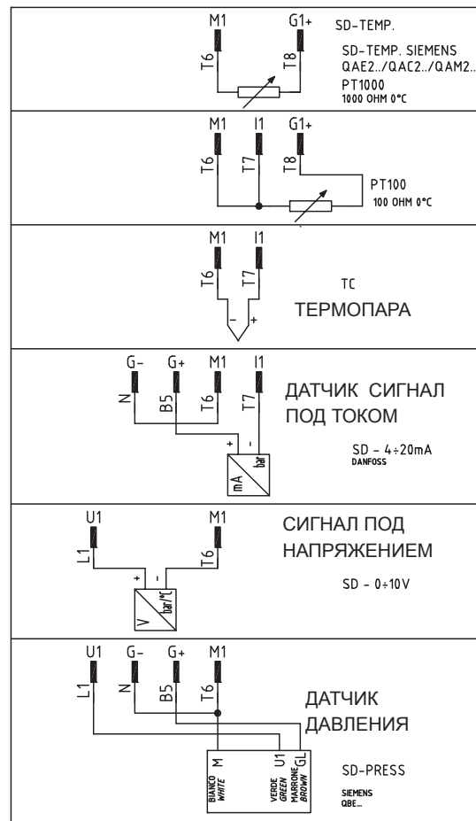
Рис. 16 - Подсоединение датчика к модулирующим горелкам
