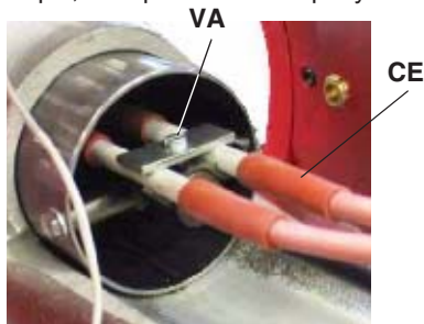
ЗАПАЛЬНЫЙ ЭЛЕКТРОДА
