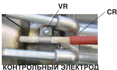
КОНТРОЛЬНЫЙ ЭЛЕКТРОД
