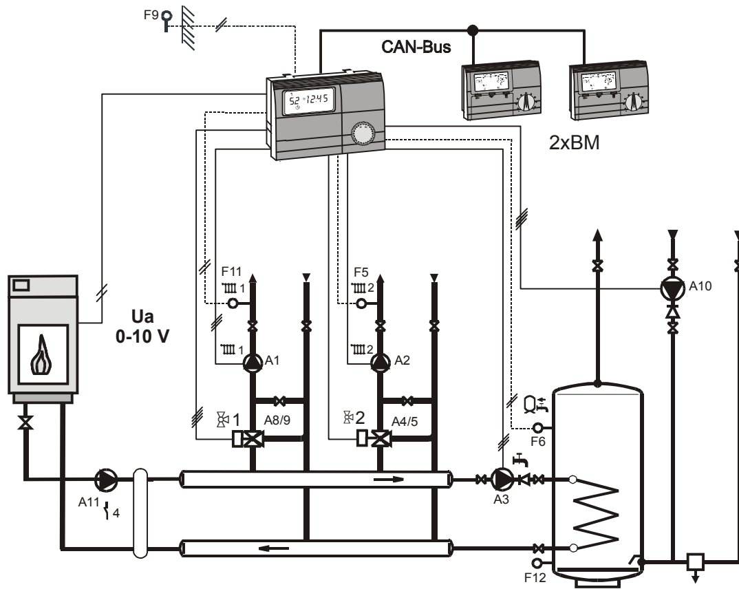
Схема 03 = E8.3611 => регулятор 0-10В
