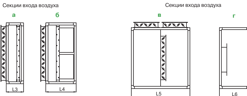
а - секция входа воздуха с кассетным фильтром G4 или F5 б - секция входа воздуха с карманным фильтром G4 или F5 (другие классы фильтров согласовываются индивидуально) в - секция разделения воздуха г - секция выравнивания воздушного потока после вентилятора
