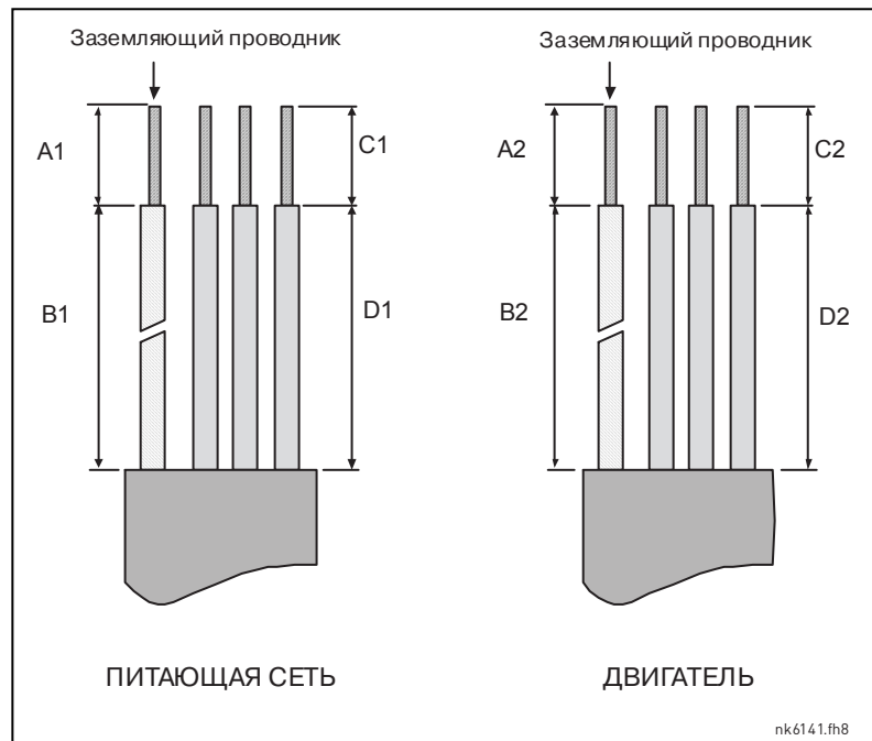
Рисунок 6-6. Зачистка кабелей
