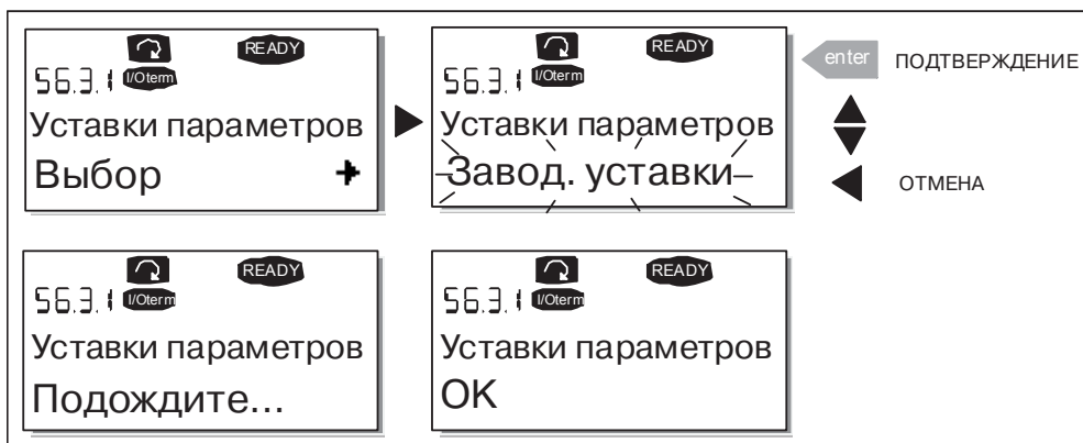
Рисунок 7-11. Сохранение и загрузка наборов параметров
