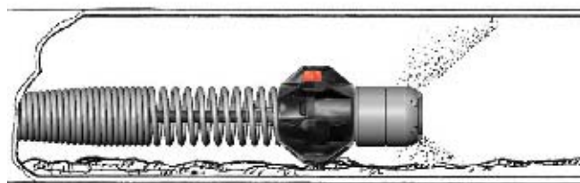
Рисунок 10 – Шаровая направляющая насадка в использовании
