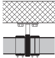
Рисунок 34: Шумопоглощающая неподвижная опора на Geberit Silent-db20 с двумя электромuftами Geberit
