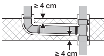
Рисунок 26: Для обеспечения заданных уровней шума толщина бетонного покрытия со всех сторон должна составлять не менее 4 см
