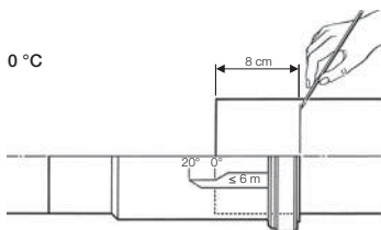
Рисунок 8: Глубина вставки компенсаторной муфты зависит от температуры
