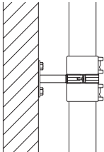
Рисунок 32: Шумопоглощающая неподвижная опора на Geberit Silent-db20 с двумя электромuftами Geberit.
