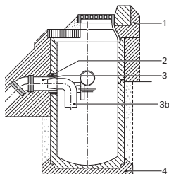
Рисунок 54: Узел соединения с колодцем
