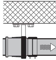
Рисунок 33: Шумопоглощающая неподвижная опора на компенсаторной муфте Geberit Silent-db20
