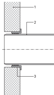
Рисунок 51: Соединение с уплотнением
