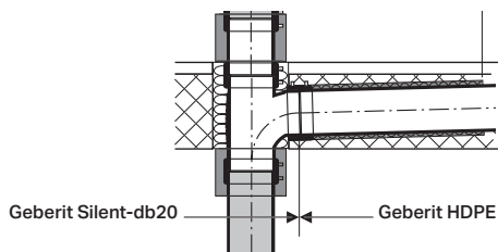
Рисунок 29: Фрагмент соединения со стояком Необходимо использовать только прямые тройники Geberit Silent-db20.
