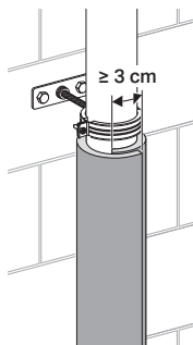
Рисунок 44:Нахлест предварительно обрезанного мата для труб Geberit Isol
