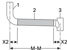
Рисунок 1: Пример расчета длины трубы
