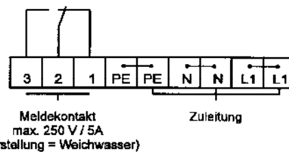
Abb. 1: Schaltplan
