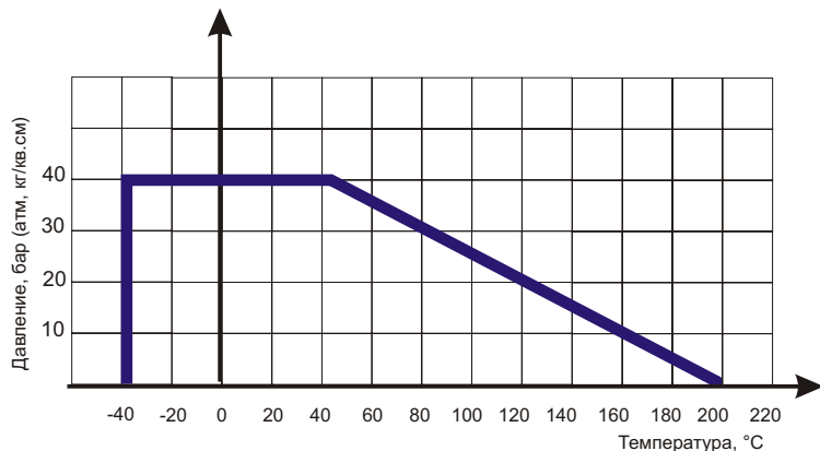
Диаграмма определяет рабочую область для шарового крана фланцевого ABRA-BV61 в координатах Давление (в барах приборного) / Температура (° C).
